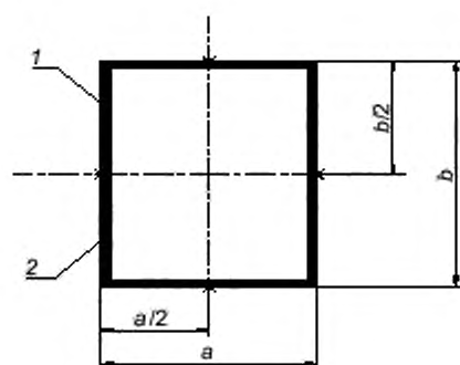
Рисунок А.4 Схема размещения TЭП на необогреваемой поверхности воздуховода
