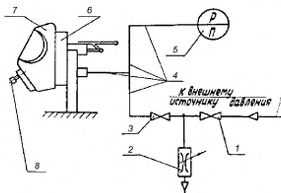
1 — запорный вентиль; 2 — дроссель; 3 — соединительный кран; 4 — соединительные трубки; 5 — мановакуумметр; 6 — герметизирующий зажим; 7 — лицевая часть; 8 — заглушка
