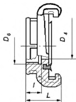
Рисунок 8 — Муфтовая всасывающая головка
