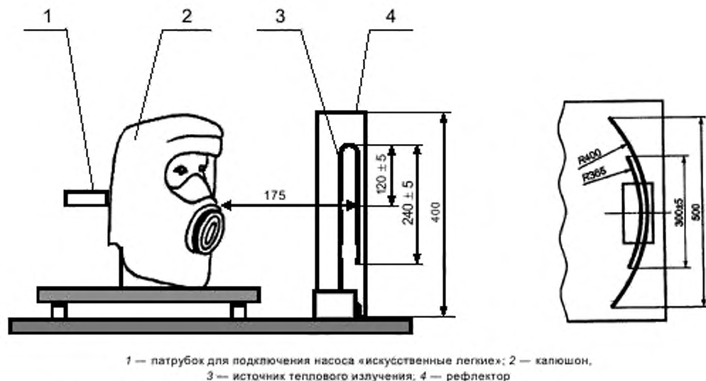
Рисунок 4 — Схема установки для определения устойчивости капюшона самоспасателя к воздействию теплового потока
