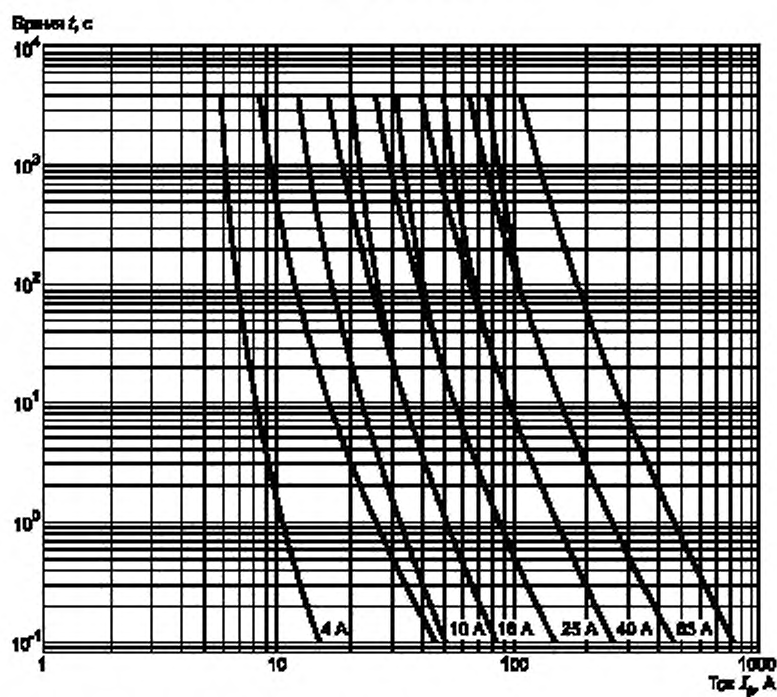
Рисунок 25b — Времятоковые зоны
