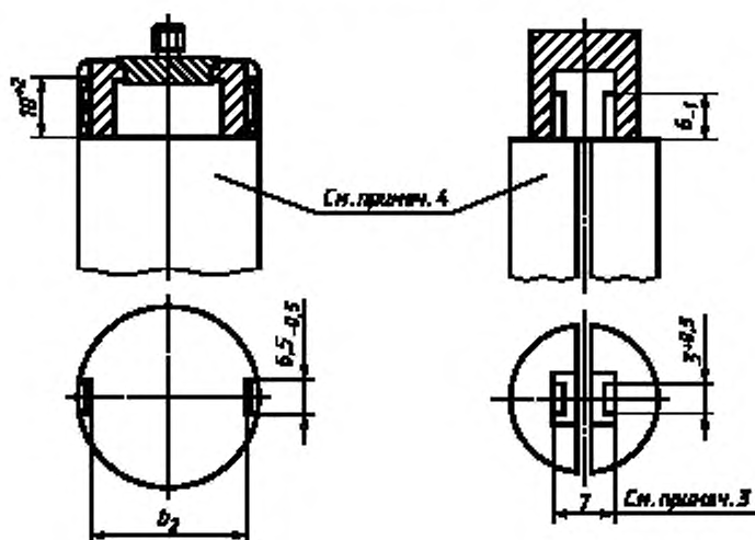
Рабочая головка ключа
