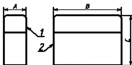
1 — держатель плавкой вставки; 2 — основание плавкого предохранителя
