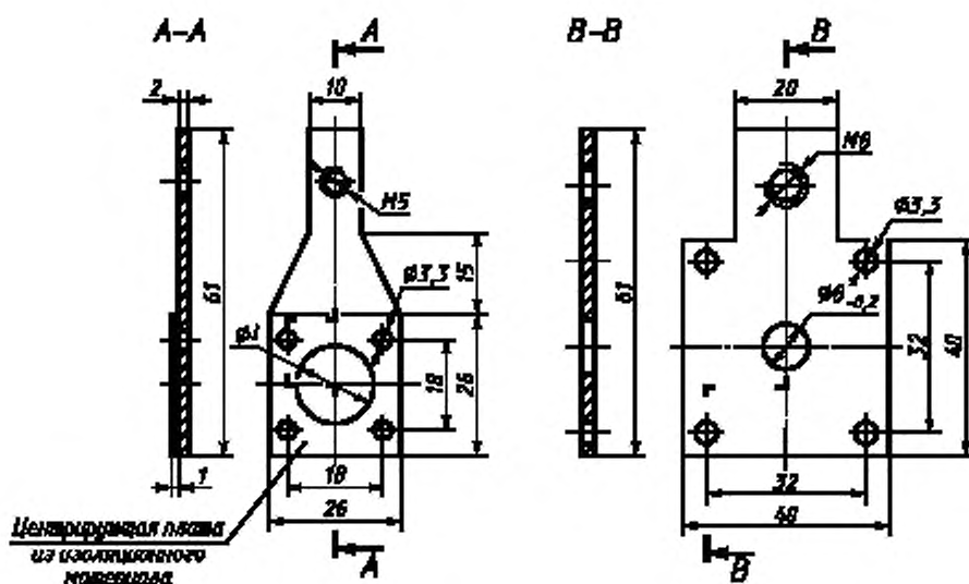
Типоразмеры D01—D03, DII, DIII
