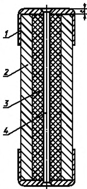
1 — колпачок; 2 — керамический корпус; 3 — наполнитель; 4 — плавкий элемент
