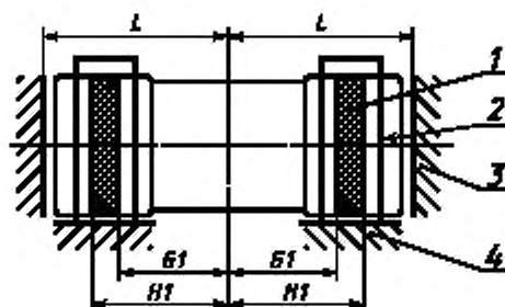
Основание типа А
