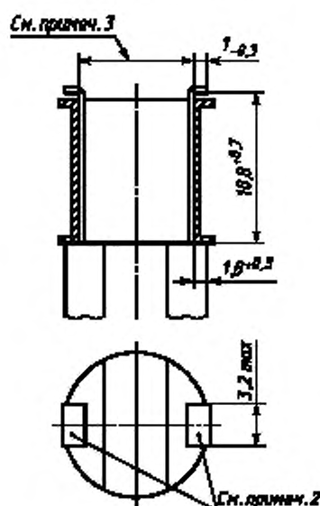
Рабочая головка ключа
