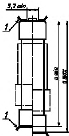
Контакты на торцевых поверхностях плавких вставок
