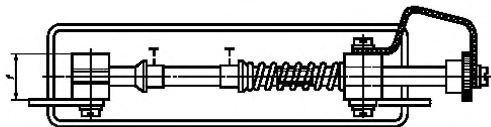
Испытательное основание
