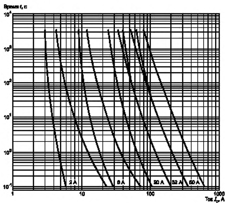
Рисунок 25a — Времятоковые зоны
