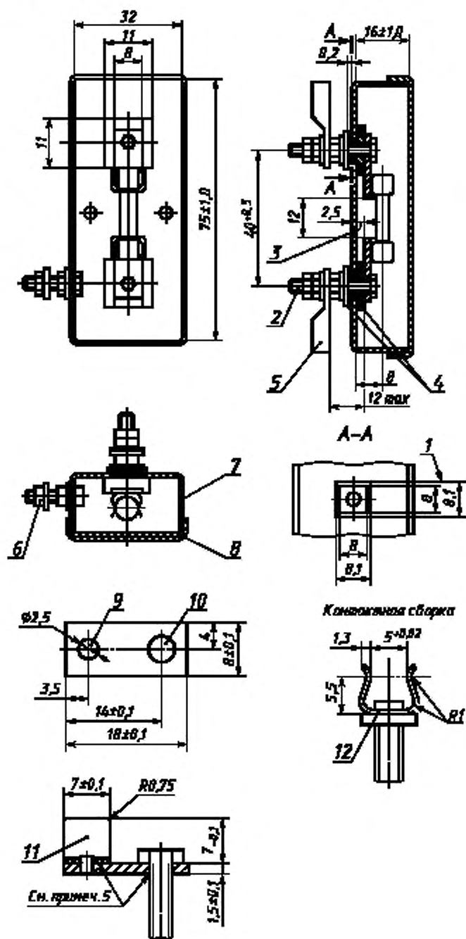
Рисунок 35 — Испытательное основание плавкого предохранителя (лист 1)
