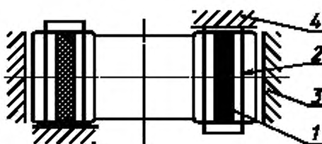
Основание типа В
