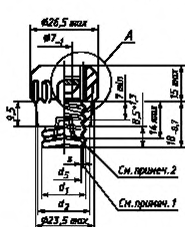
Типоразмеры D01, D02
