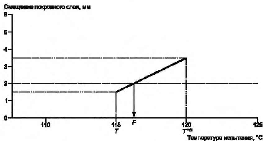
Рисунок 2 — Пример определения предельного значения теплостойкости интерполяцией
