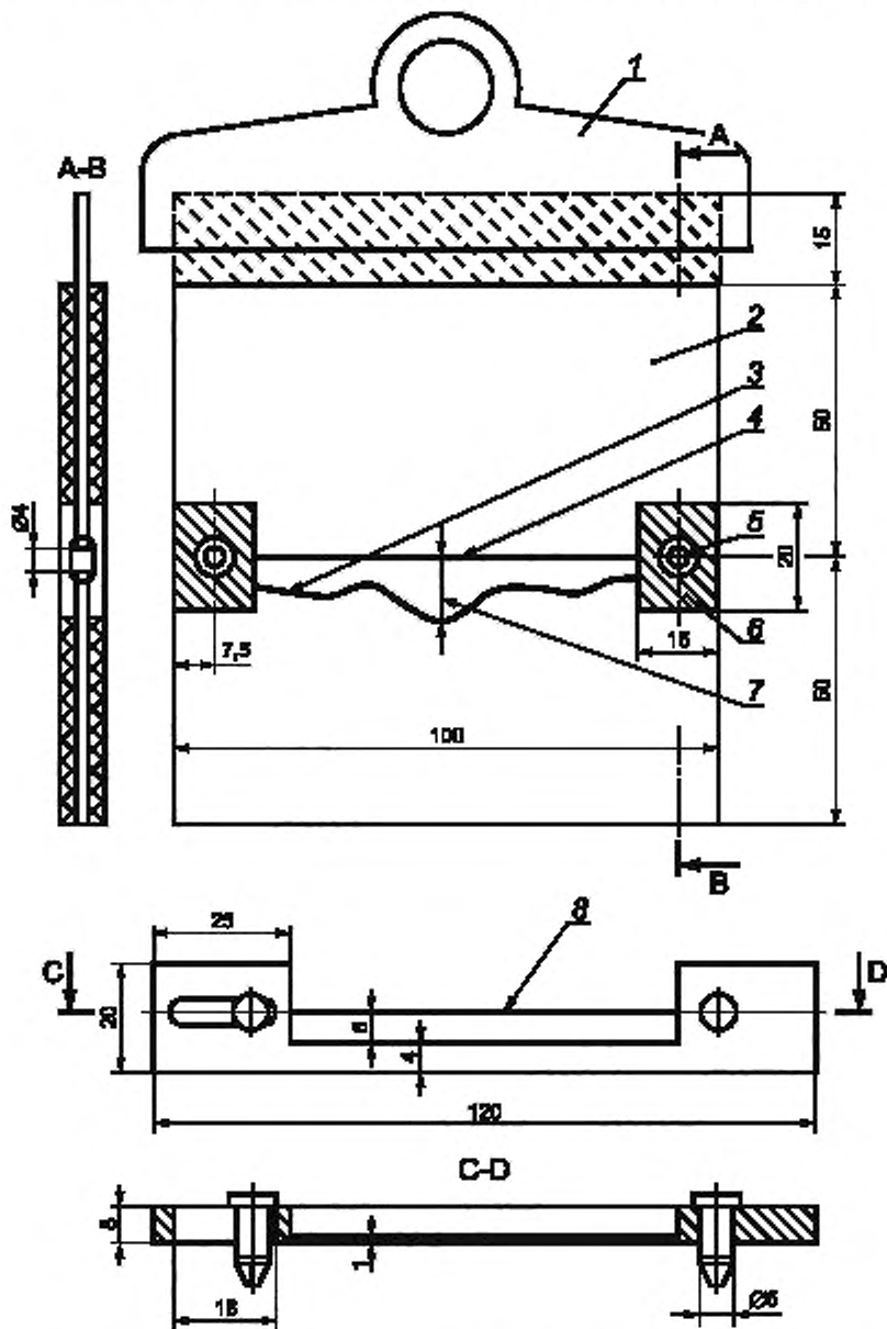
1 — приспособление для подвешивания образца; 2 — образец; 3 — маркировочная линия 1; 4 — маркировочная линия 2; 5 — металлический поршень с внутренним диаметром 4 мм; 6 — участок с удаленным покровным слоем; 7 — максимальное расстояние между маркировочными линиями \Delta l ; 8 — прямая кромка
