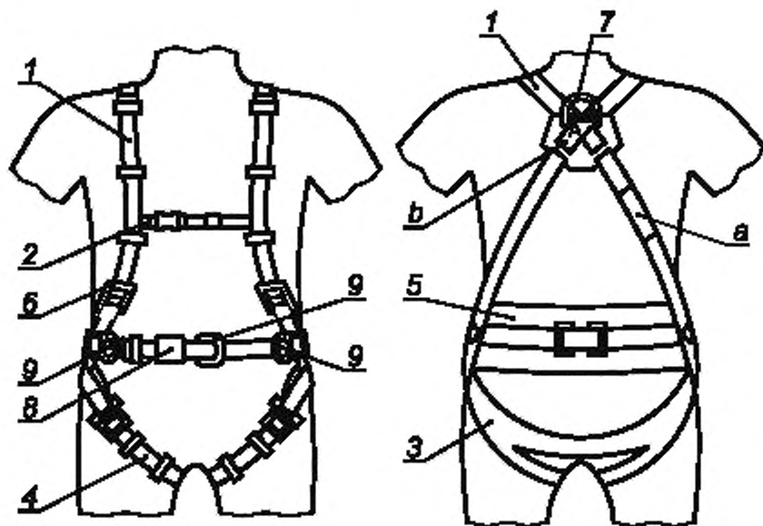
1 — наплечная ляжка; 2 — вспомогательная ляжка; 3 — ремень, используемый в положении сидя; 4 — набедренный ремень; 5 — спинная опора для рабочего позиционирования; 6 — регулировочный элемент; 7 — элемент крепления для останова падения; 8 — пряжка; 9 — элемент крепления для рабочего позиционирования;
