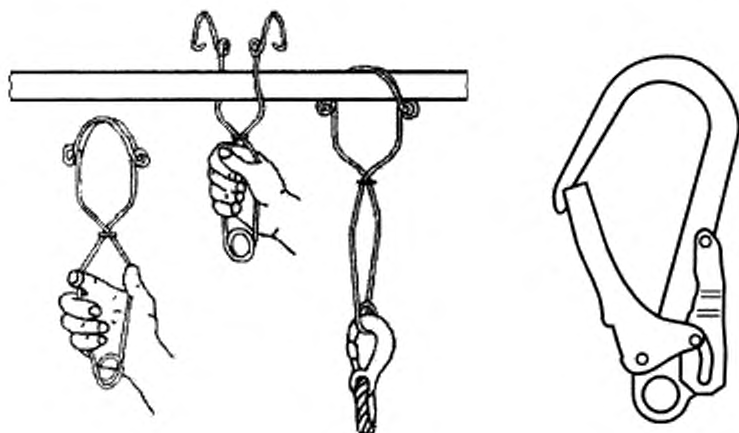
Рисунок 3 — Пример анкерных соединительных элементов (класс А)
