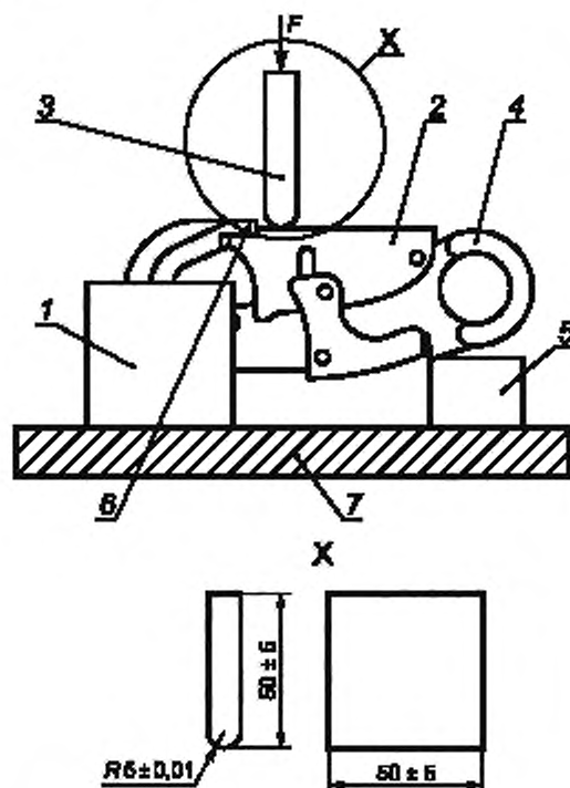
1 — зажимное приспособление; 2 — запорный элемент; 3 — нагрузка (жесткий стержень); 4 — соединительный элемент; 5 — опорный блок (альтернативно круглый стержень в проушине); 6 — носовая часть; 7 — испытательный стенд
