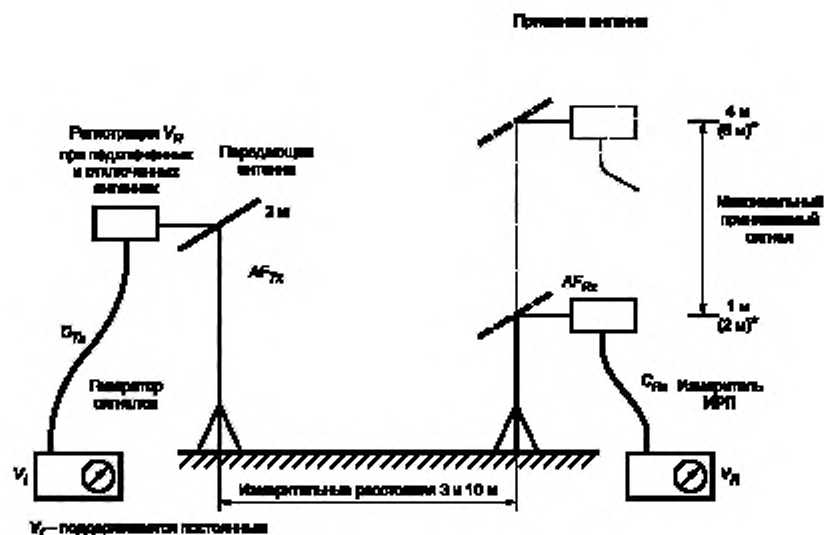
Рисунок 4 — Расположение оборудования для измерения затухания площадки при горизонтальной поляризации (см. 5.6 и приложение Е)
