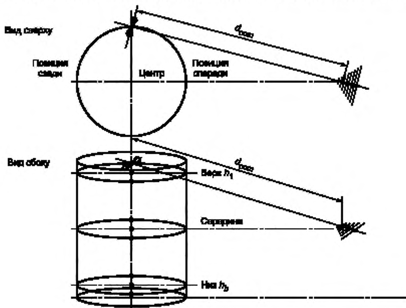
Рисунок 9 — Пример одной из измерительных позиций и наклона антенны при процедуре валидации измерительной площадки
