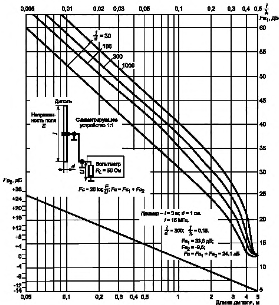
Рисунок 1 — Градуировочные коэффициенты коротких дипольных антенн при R_L = 50 \text{ Ом}
