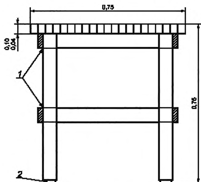
Рисунок А.1 — Испытательный стол
