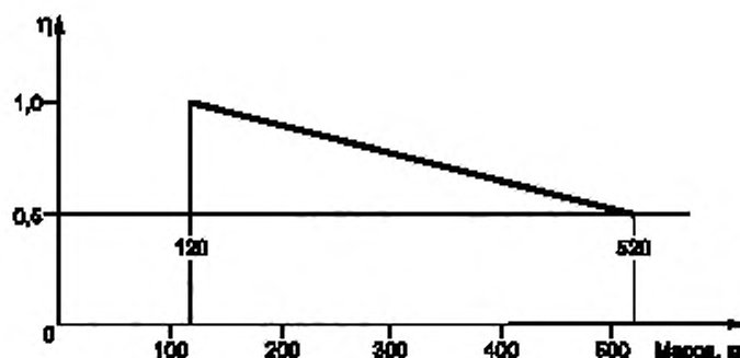
Рисунок 5 — Спектральный коэффициент нагрузки \eta
