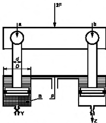
В — нагрузка, вызывающая продольный изгиб; F — нагрузка; p — давление в системе; P_{FC} — нормальное давление; Z — ограниченный расход; Y — заблокированная линия
