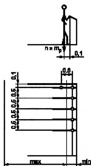
Рисунок 2 — Номинальная нагрузка (масса людей)
