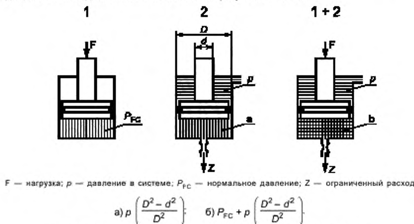
Рисунок F.1 — Давление в цилиндре при обычном режиме работы (цилиндр работает на сжатие)
