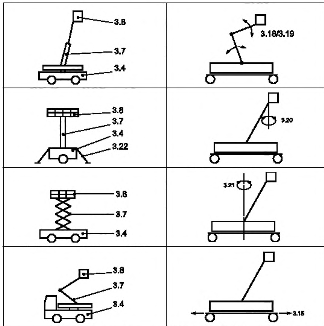
Рисунок 1 — Примеры к определениям 3.4, 3.7, 3.8, 3.15, 3.18, 3.19, 3.20, 3.21, 3.22
