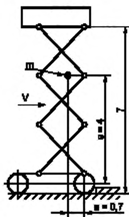
Рисунок С.1 — МПРП перед препятствием
