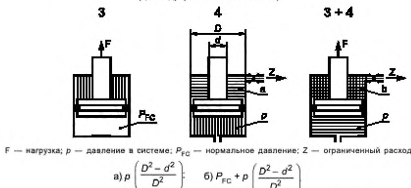
Рисунок F.2 — Давление в цилиндре при обычном режиме работы (цилиндр работает на растяжение)
