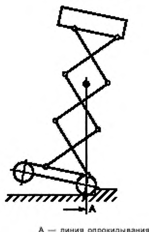
Рисунок С.2 — МПРП у препятствия
