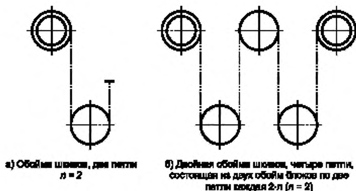
Рисунок D.3 — Обоймы блоков
