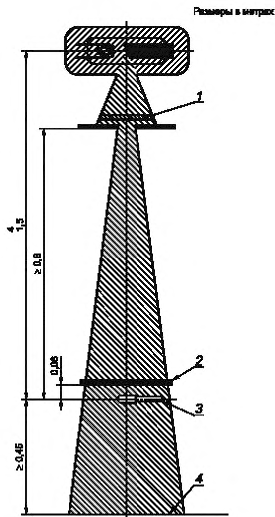
Рисунок 6 — Геометрическая схема устройства для измерения чувствительности (способы экспонирования I, II и III)
