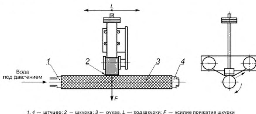
Рисунок 3 — Схема истребления образца рукава
