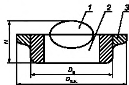
1 — запирающий элемент; 2 — проходное отверстие; 3 — фланец пришивного кольца, H — высота ПКС, D_{\text{п}} — посадочный диаметр ПКС; D_{\text{п.н.}} — пришивной наружный диаметр ПКС
