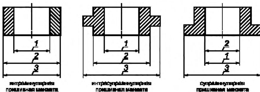
Рисунок 2 — Типы пришивных манжет
