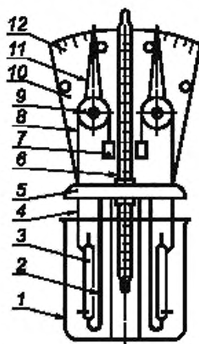
1 — стакан; 2 — неподвижный крючок; 3 — образец кожаной ткани; 4 — подвижной крючок; 5 — металлическая пластина; 6 — термометр; 7 — груз; 8 — прочная нить; 9 — шкив; 10 — вертикальная стойка; 11 — подвижная стрелка; 12 — шкала
