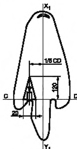
Рисунок 5 — Схема расположения образцов на шкурках, выделанных трубкой для химических анализов и определения температуры сваривания (Т)
