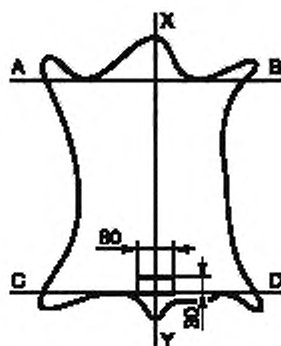
Рисунок 3 — Схема расположения образцов для определения светостойкости окраски
