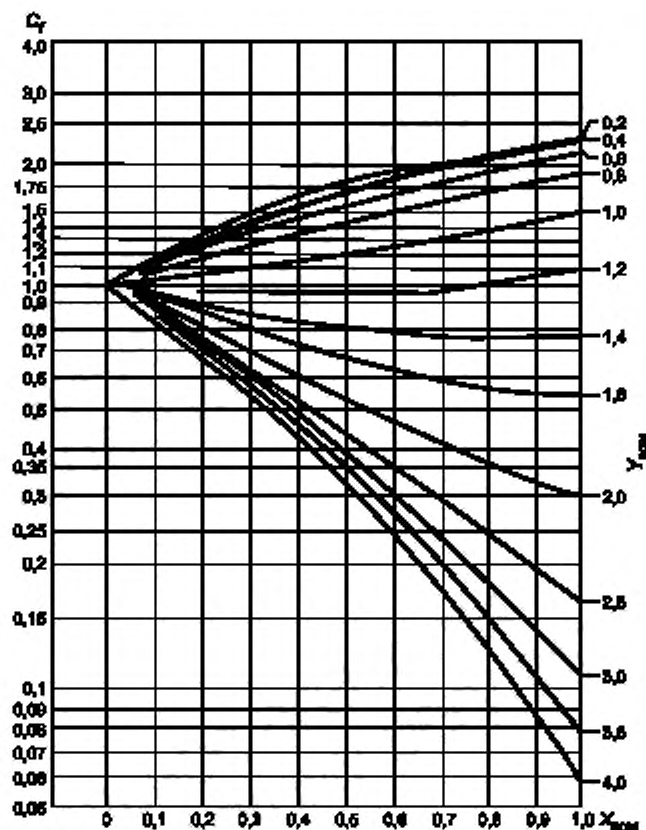
Рисунок 25 — Параметр жесткости компенсатора C_f
