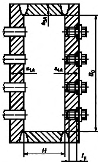
Рисунок 21 — Сварная камера без перегородок
