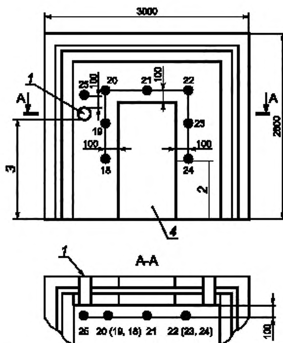
1 — вход кабеля, 2 — половина высоты двери; 3 — 2/3 внутренней высоты испытываемого образца; 4 — дверь
