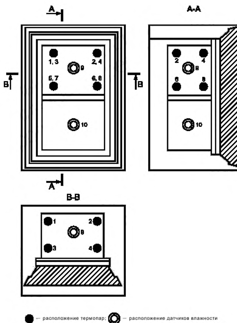
Рисунок 6 — Точки измерений (1—10) в испытываемых образцах контейнеров данных
