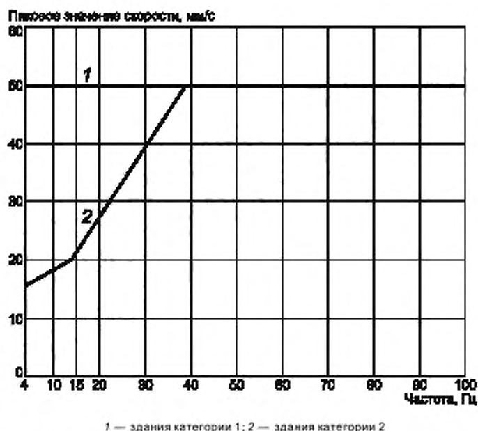
Рисунок Б.2 — Предельные значения скорости, измеренной на фундаменте здания
