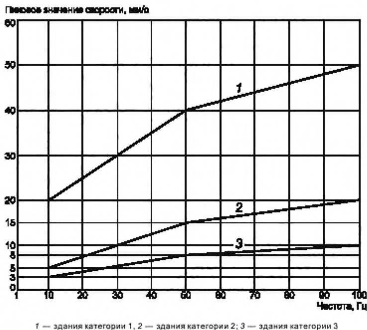
Рисунок Б.1 — Предельные значения скорости, измеренной на фундаменте здания
