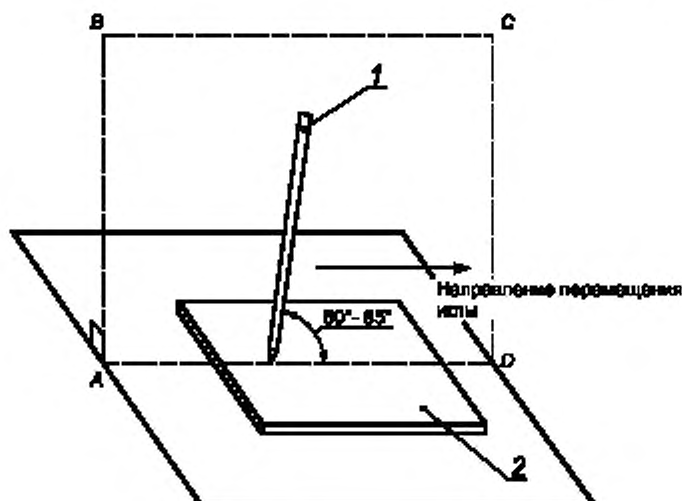
1 — игла; 2 — испытуемый образец
