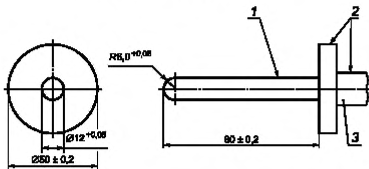
Рисунок 2В — Испытательный штырь
