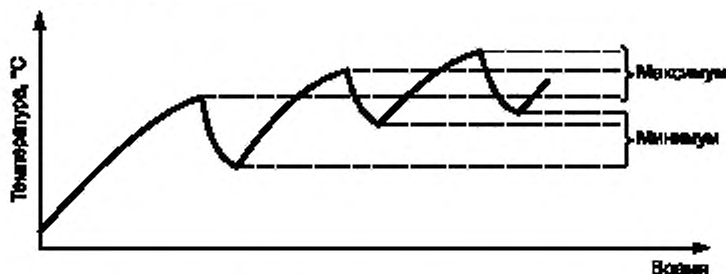
Рисунок С.1 — Определение среднееарифметического значения температуры
