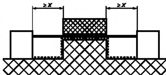
Рисунок F.5 — Несплошной стык с узкими канавками
