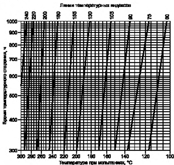
Рисунок 2G — Время теплового старения
