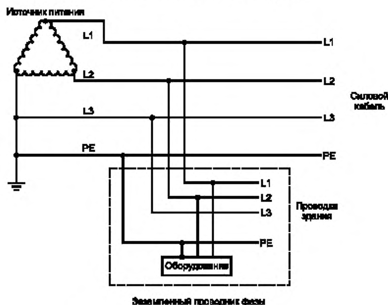
Рисунок V.1 — Пример TN-S-системы электропитания
