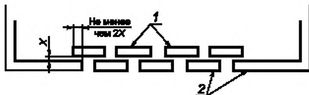
Рисунок 4F — Конструкция отражающей пластины
