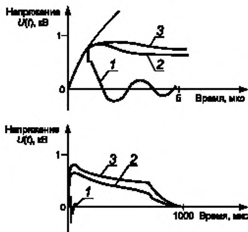
Рисунок S.3 — Форма сигнала при работающем ограничителе перенапряжений
