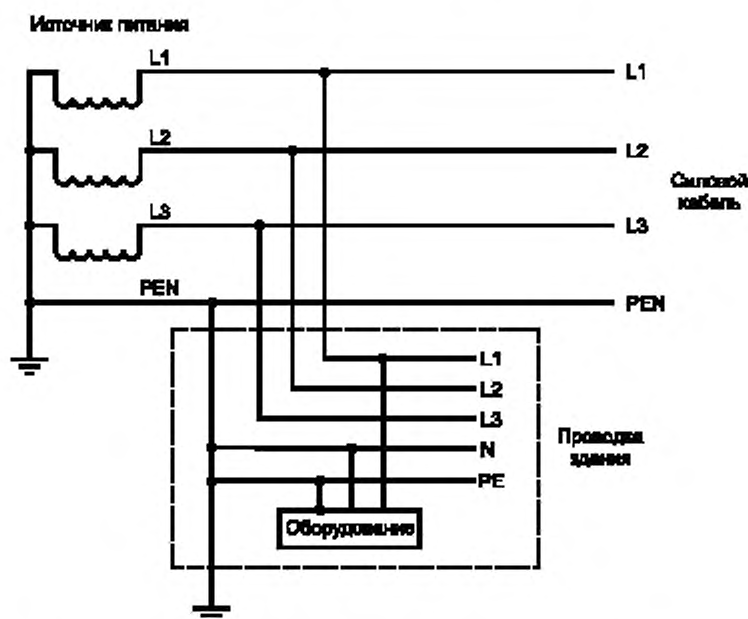
Рисунок V.2 — Пример TN-C-S-системы электропитания
