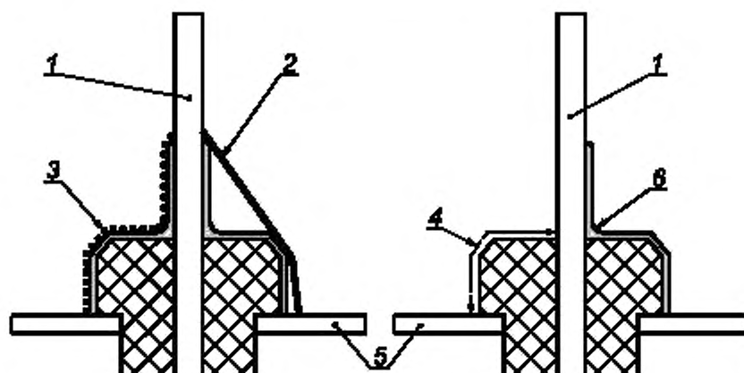
Рисунок F.9 — Широкое углубление
