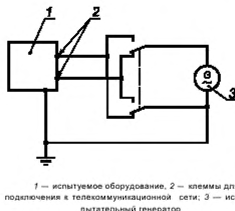
Рисунок 2E — Испытательный генератор
