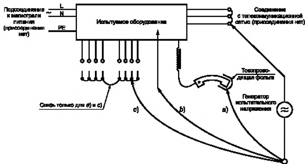
Рисунок 6B — Точки приложения испытательного напряжения
