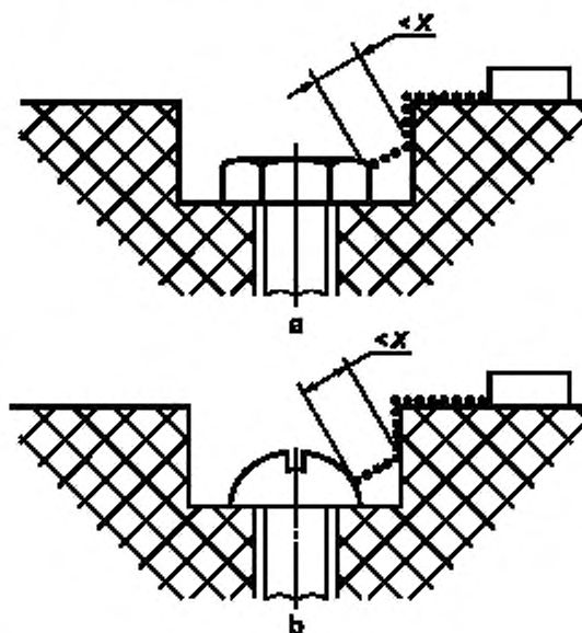
Рисунок F.7 — Неплотный стык с узкой и широкой канавками
