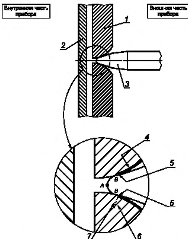
1 — кожух из изоляционного материала; 2 — часть цели СИН или часть, находящаяся под опасным напряжением; 3 — испытательный палец; 4 — поверхность, считающаяся покрытой металлической фольгой; 5 — точка контакта; 6 — доступная для испытательного пальца поверхность; 7 — недоступная для испытательного пальца поверхность
