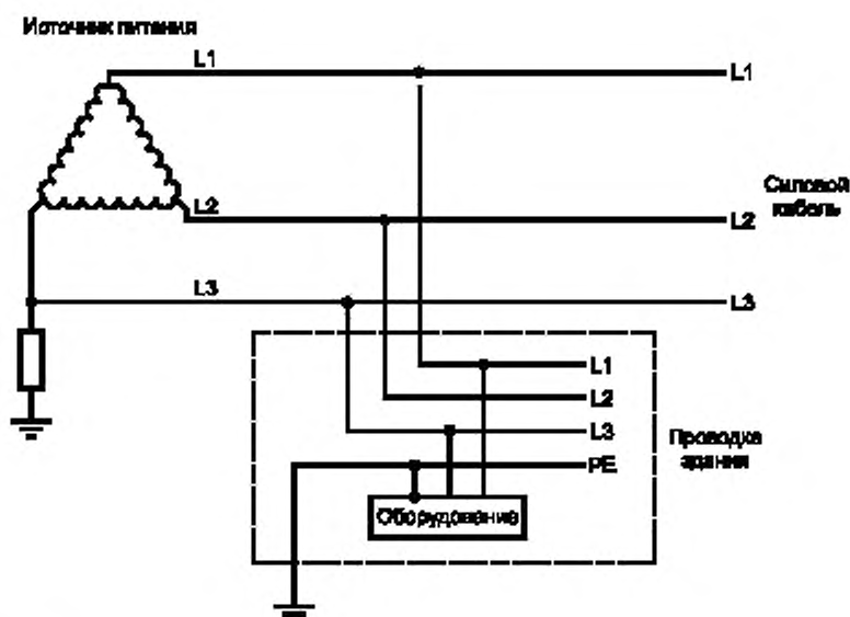
Рисунок V.8 — Пример IT-системы электропитания с тремя фазами
