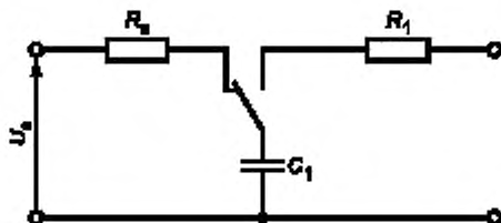
Рисунок N.2 — Схема испытательного генератора импульсов по МЭК 60065
