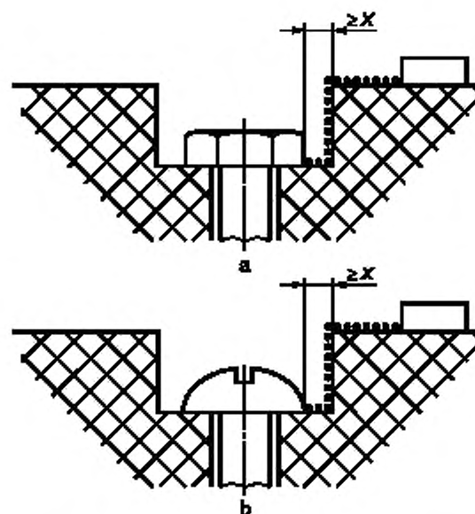
Рисунок F.9 — Широкое углубление
