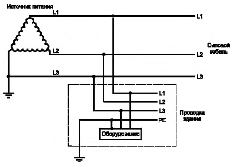
Рисунок V.6 — Пример TT-системы электропитания с тремя фазами
