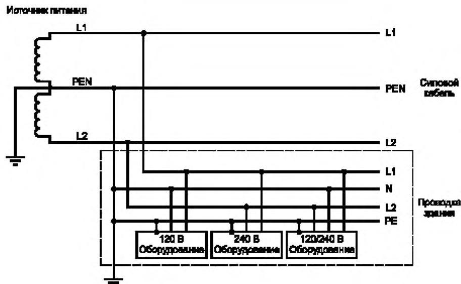
Рисунок V.4 — Пример однофазной трехпроводной TN-C-системы электропитания
