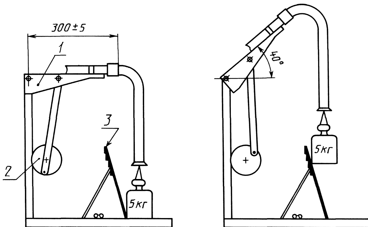
1 — качающийся рычаг; 2 — кривошипный механизм; 3 — наклонная плоскость
