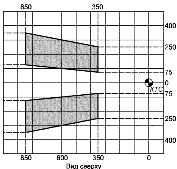
Рисунок 3 — Зоны расположения педалей двустороннего действия
