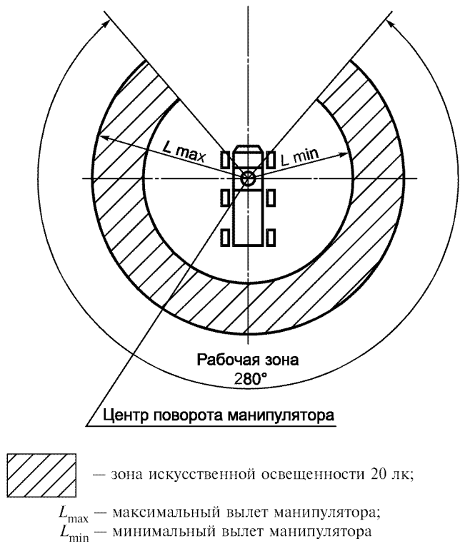
Рисунок Б.5 — Погрузочно-транспортные машины
