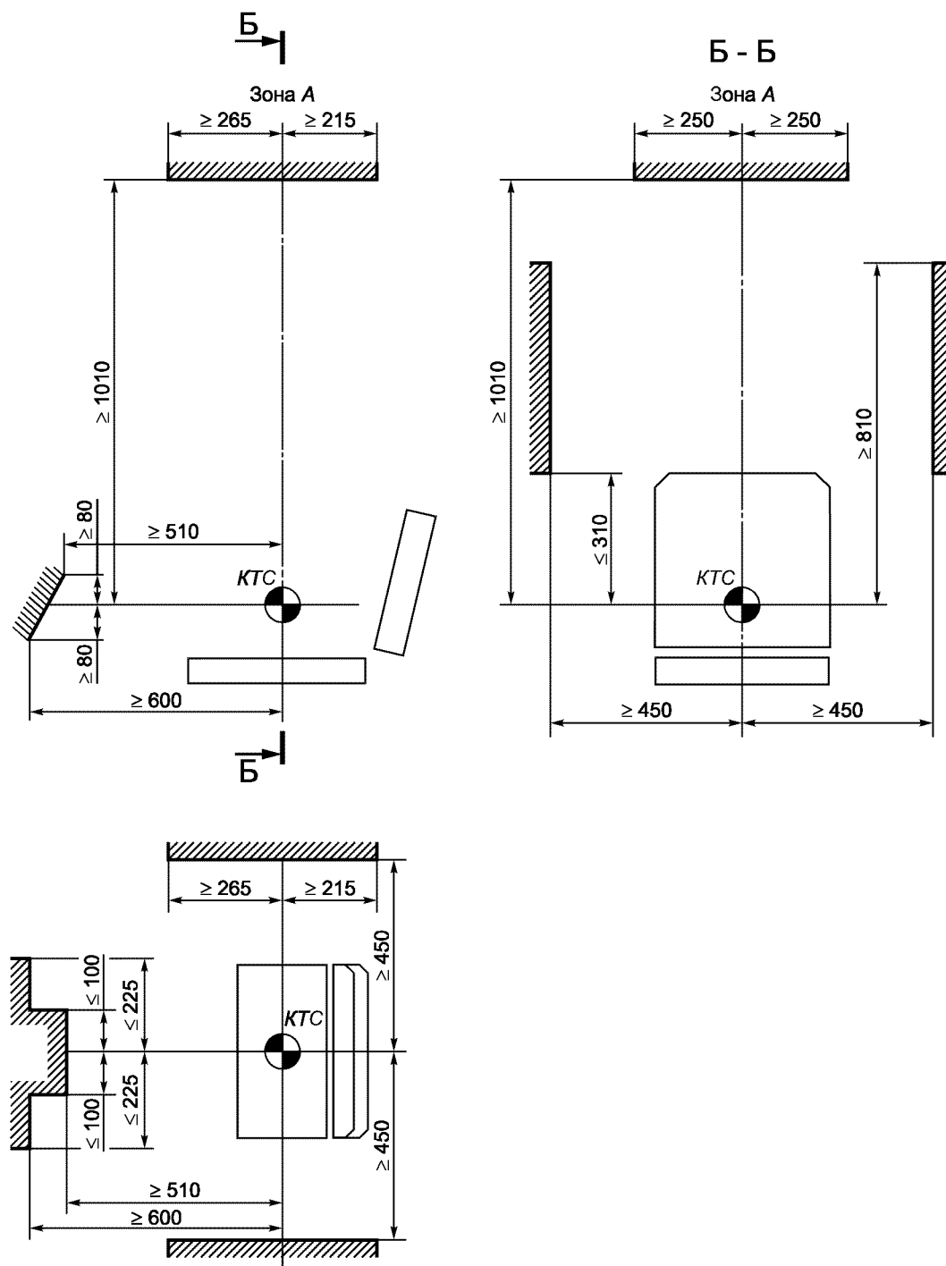
Рисунок 1 — Размеры минимального рабочего пространства для машин с реверсивным постом управления
