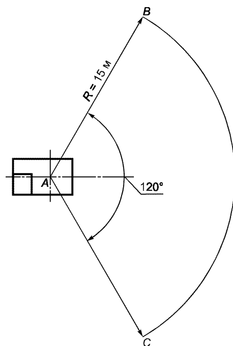
Рисунок Б.2 — Трелевка леса бесчокерная
