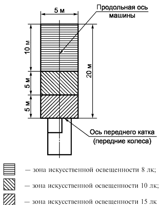
Рисунок Б.7 — Участок лесосеки, волока, дороги при движении машины
