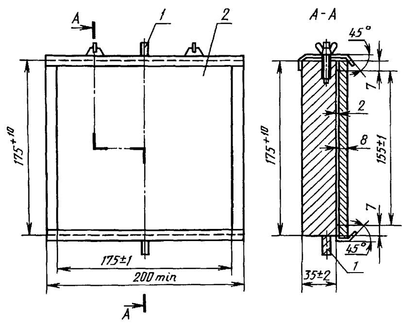
1 — шарнир; 2 — лист фанеры
