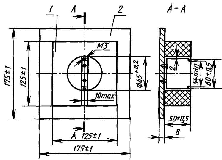
1 — брусок из граба; 2 — лист фанеры
