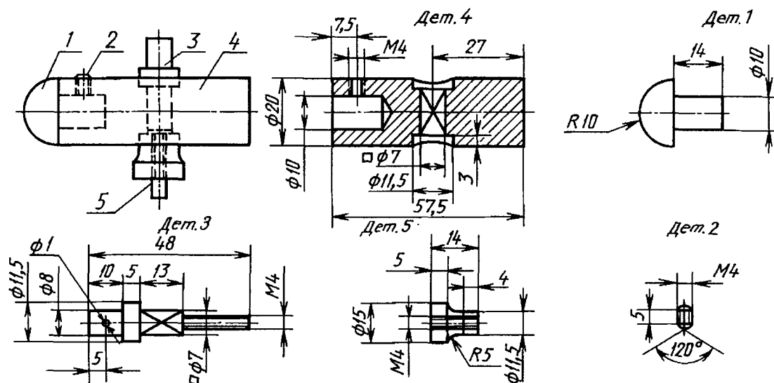
Материал деталей: 1 — полиамид; 2— 5 — сталь
