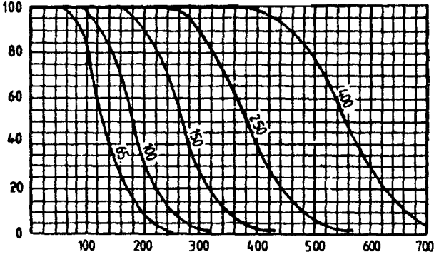
График D — Кривые оперативных характеристик для одноступенчатых планов (кривые двух- и многоступенчатого контроля по возможности максимально близки)
