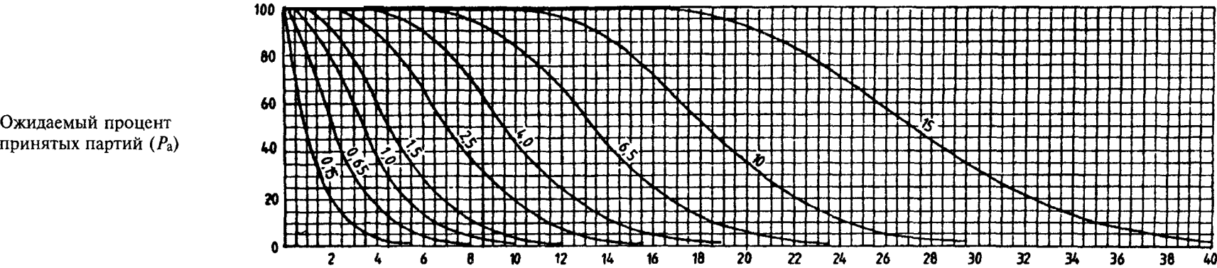
График J — Кривые оперативных характеристик для одноступенчатых планов (кривые двух- и многоступенчатого контроля по возможности максимально близки)
