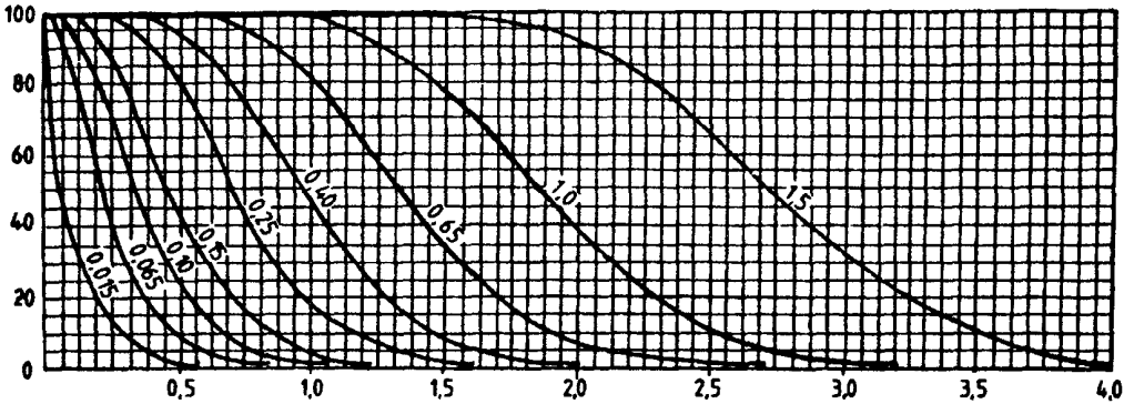
График Р — Кривые оперативных характеристик для одноступенчатых планов (кривые двух- и многоступенчатого контроля по возможности максимально близки)
