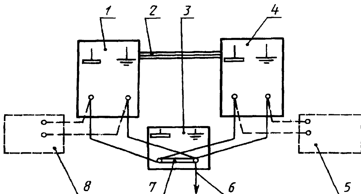
1 — первая стойка испытуемого ТС АС-ЯРО; 2 — линии связи между стойками; 3 — опорный узел заземления ТС АС-ЯРО; 4 — n -я стойка испытуемого ТС АС-ЯРО; 5 — подключение ИГ к n -й стойке испытуемого ТС АС-ЯРО; 6 — цепь связи с физической землей; 7 — переключатель между сигнальной и защитной системами заземления; 8 — подключение ИГ к первой стойке испытуемого ТС АС-ЯРО
