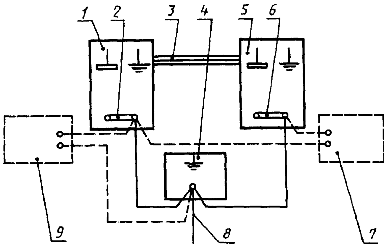
1 — первая стойка испытуемого ТС АС-ЯРО; 2, 6 — перемычки между сигнальной и защитной системами заземления в стойке; 3 — линии связи между стойками; 4 — опорный узел заземления ТС АС-ЯРО; 5 — n-я стойка испытуемого ТС АС-ЯРО; 7 — подключение ИГ к зажимам защитного заземления двух стоек; 8 — цепь связи с физической землей; 9 — подключение ИГ к зажиму защитного заземления стойки и к опорному узлу заземления
