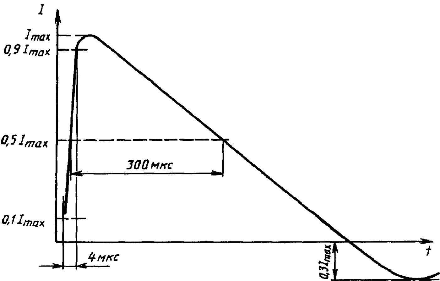
Рисунок 5 — Форма импульса тока на короткозамкнутом выходе ИГ
