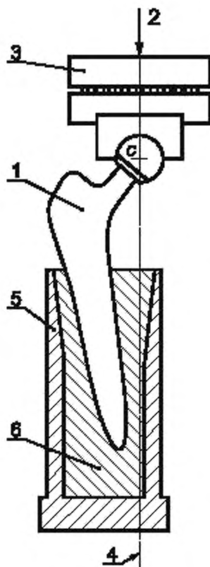
Рисунок 1 — Общий вид расположения испытуемого образца
