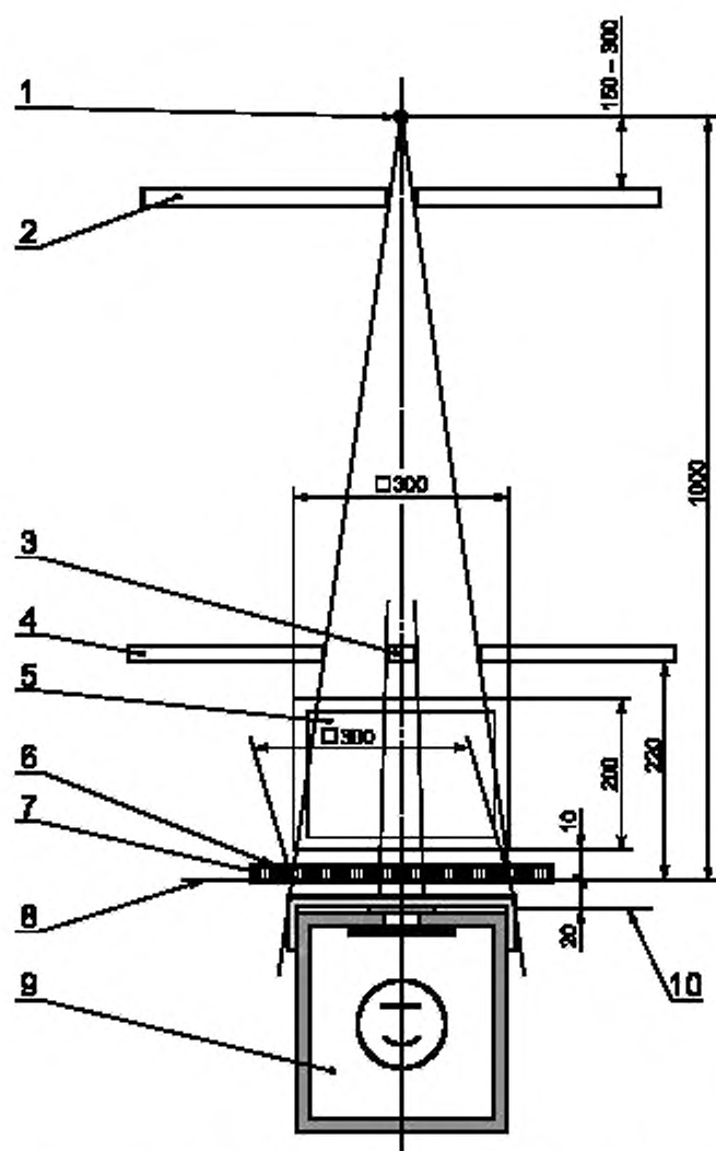
1 — ФОКУСНОЕ ПЯТНО; 2, 4 — ДИАФРАГМА; 3 — свинцовый экран для ПЕРВИЧНОГО ИЗЛУЧЕНИЯ; 5 — ФАНТОМ; 6 — входная поверхность; 7 — ОТСЕИВАЮЩИЙ РАСТР; 8 — плоскость держателя; 9 — ДЕТЕКТОР ИЗЛУЧЕНИЯ; 10 — выходная плоскость ЛЮМИНЕСЦЕНТНОГО ЭКРАНА
