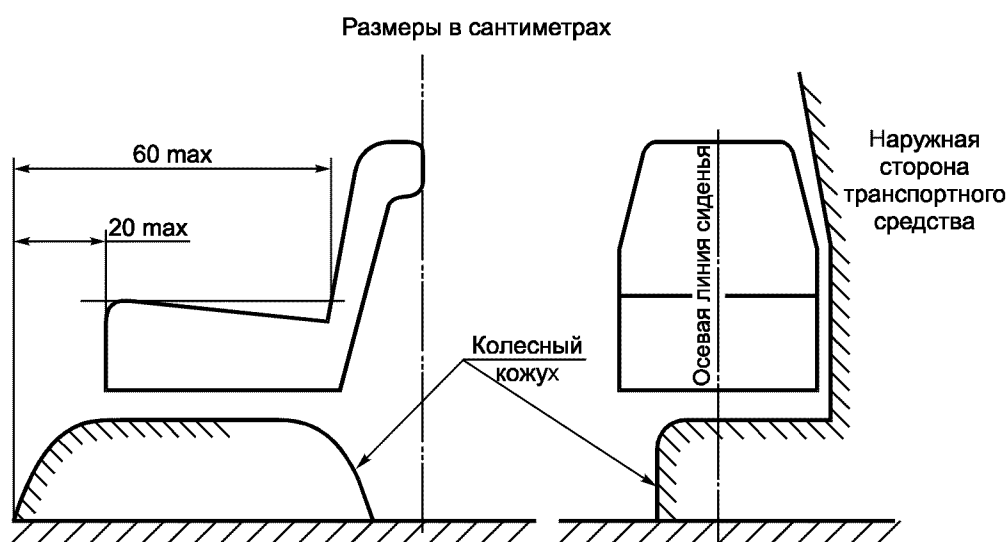
Рисунок 10 — Допустимое расположение колесного кожуха, выступающего за вертикальную осевую линию бокового сиденья (см. 5.7.8.1.3.4)
