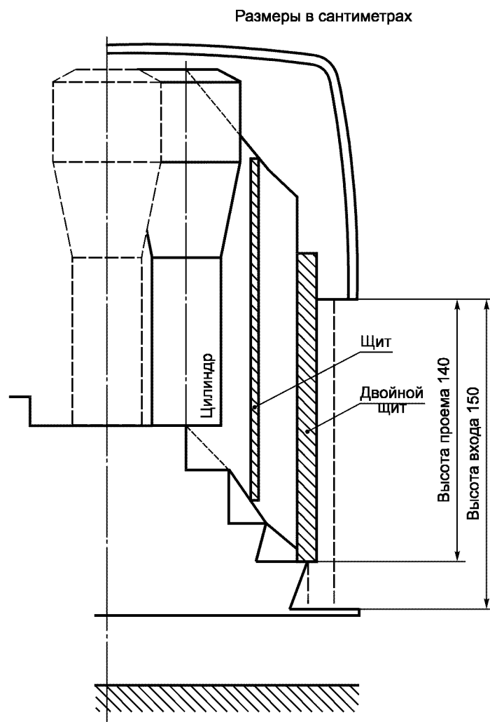
Рисунок 17 — Служебная дверь (см. 5.7.1.4)
