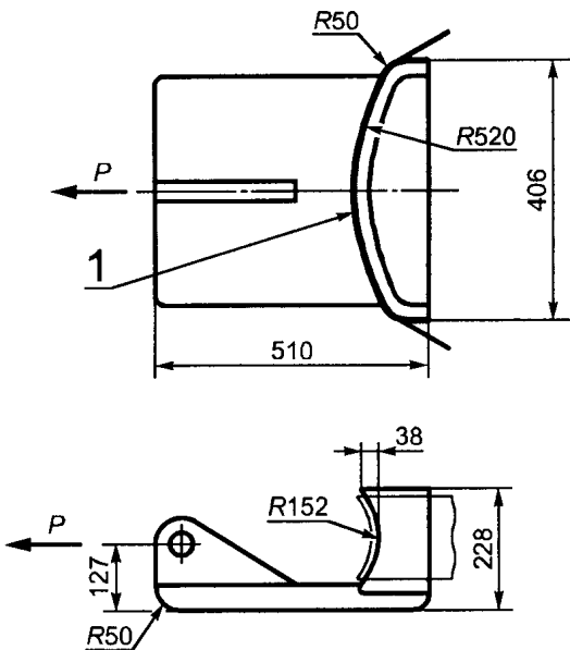
1 — пористый материал, покрытый полотном, толщина 25 мм; P — испытательная нагрузка
