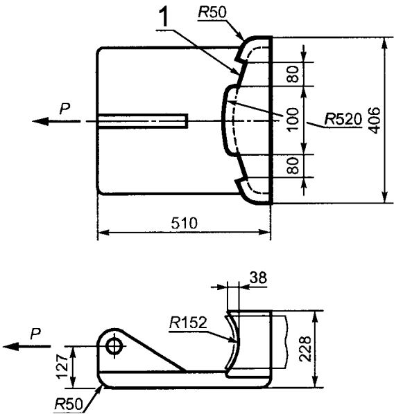
1 — пористый материал, покрытый тканью, толщина 25 мм; P — испытательная нагрузка
