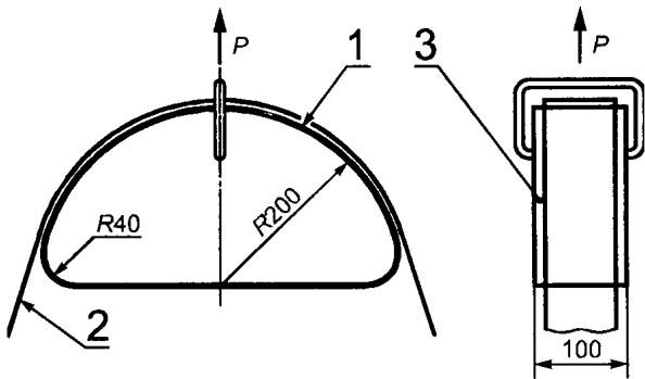
1 — пористый материал, покрытый полотном, толщина 25 мм; 2 — лямка, связывающая блок с точками крепления; 3 — блок; P — испытательная нагрузка
