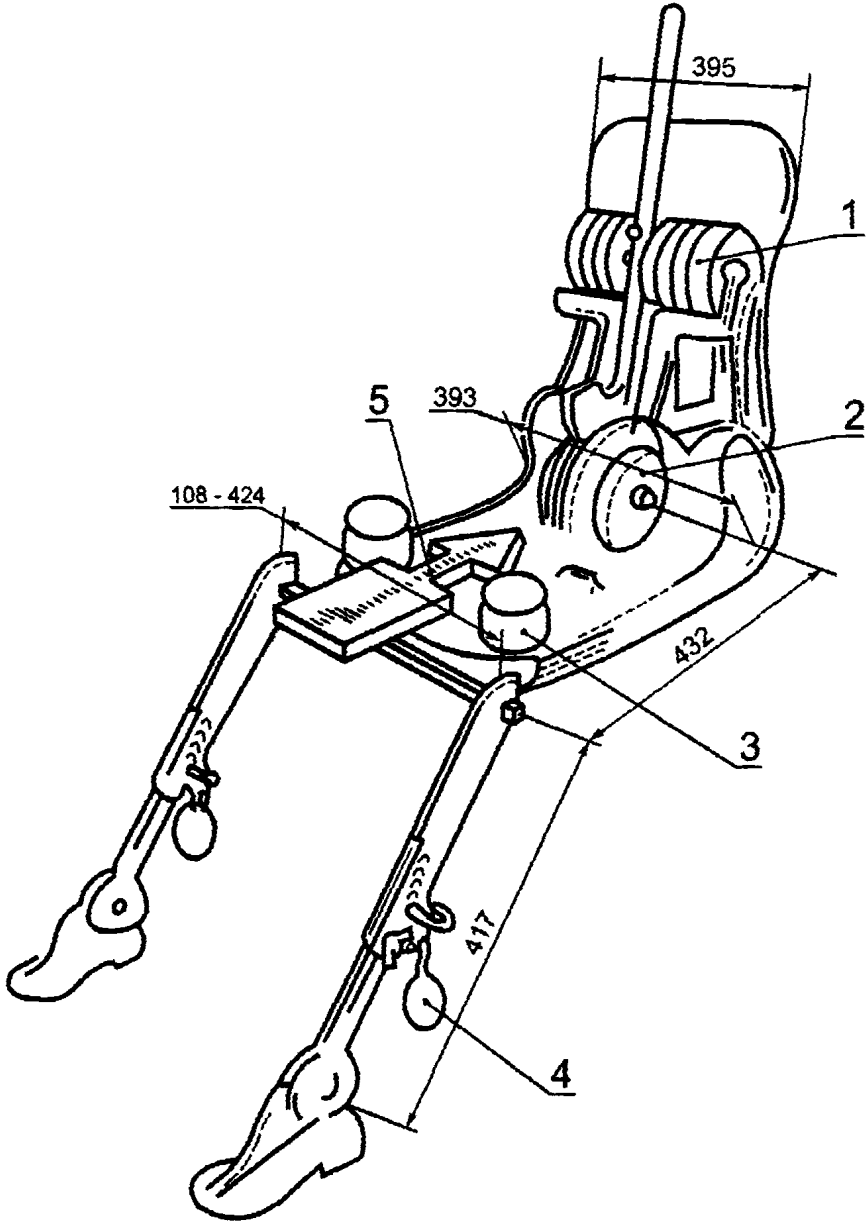
1 — спинные грузы; 2 — сидалищные грузы; 3 — набедренные грузы; 4 — ножные грузы
