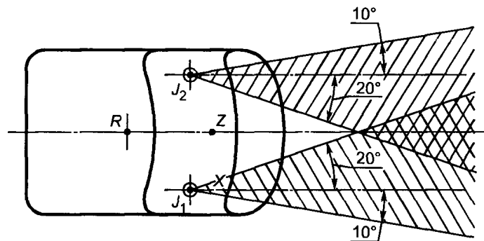
Рисунок 2 — Верхние точки эффективного крепления ремня, соответствующие 5.4.3.7.3
