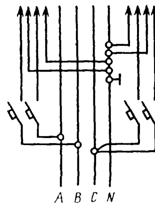
Черт. 3
