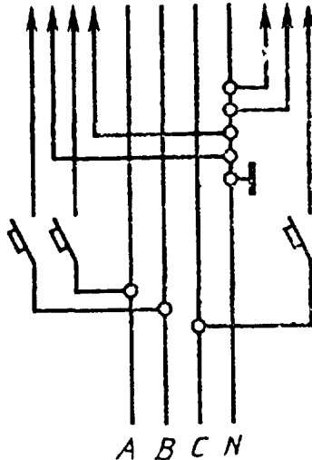
Черт. 2
