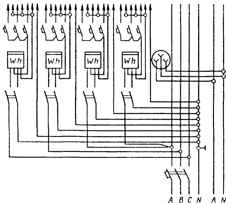
Черт. 6
