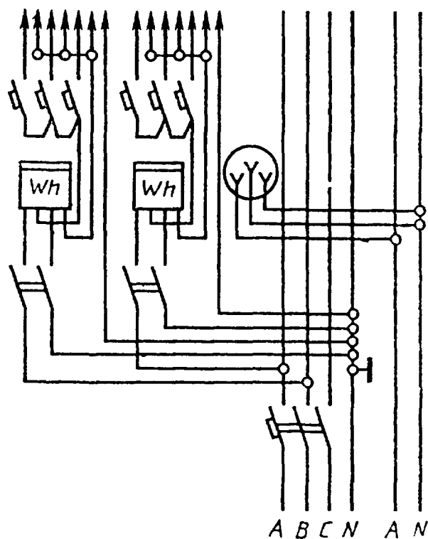
Черт. 4
