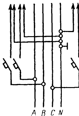
Черт. 2
