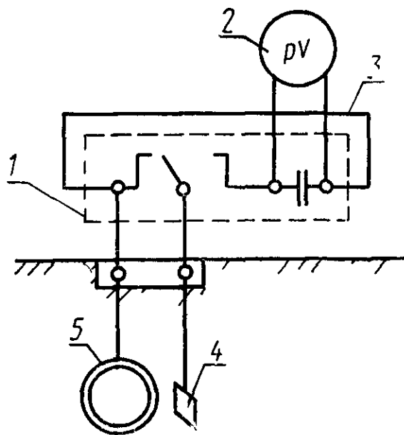
Принципиальная схема определения полярности омического падения потенциала
