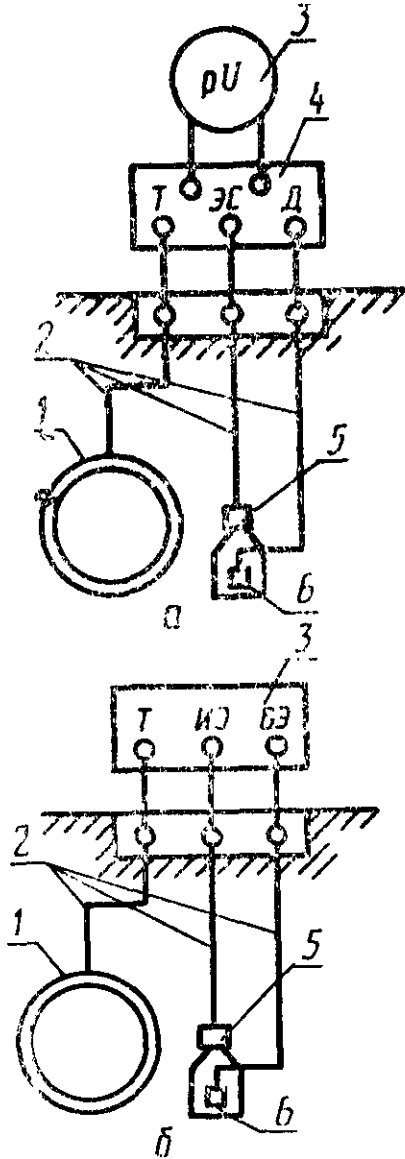
1—трубопровод; 2—контрольные проводни- ки; 3—вольтметр; 4—прерыватель тока; 5—медисульфатный электрод сравнения; 6—датчик потенциала
