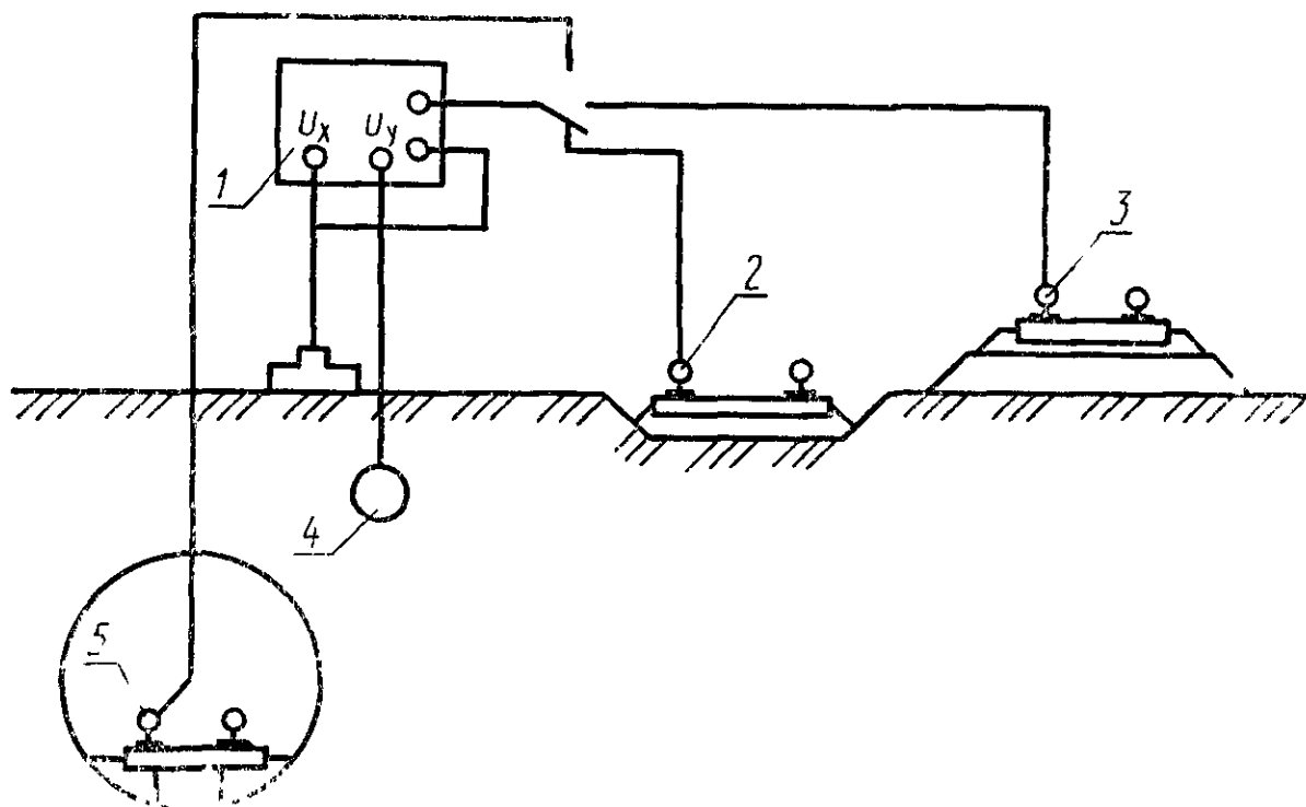
1—графопостроитель; 2—рельсы трамвая; 3—рельсы железной дороги; 4—подземное сооружение; 5—рельсы метрополитена
