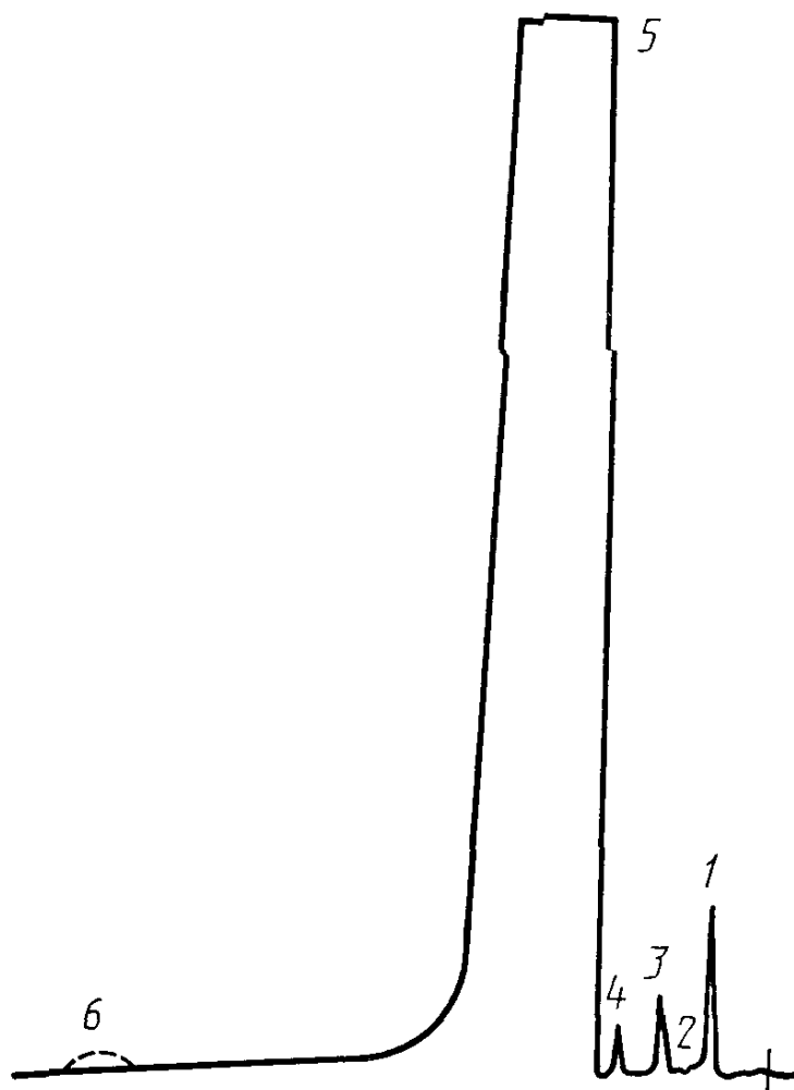
Типовая хроматограмма хладона 22
