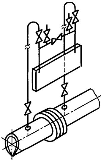
Рисунок В.1 — Дифманометр над трубопроводом
