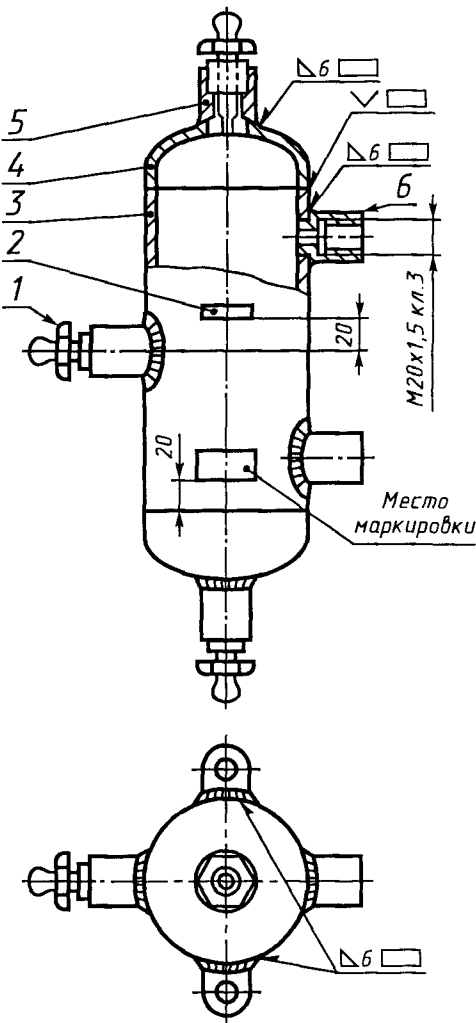
1 — пробка; 2 — ушко; 3 — обечайка; 4 — дно; 5 — штуцер; 6 — штуцер Рисунок 8— Конструкция разделитель- ного сосуда
