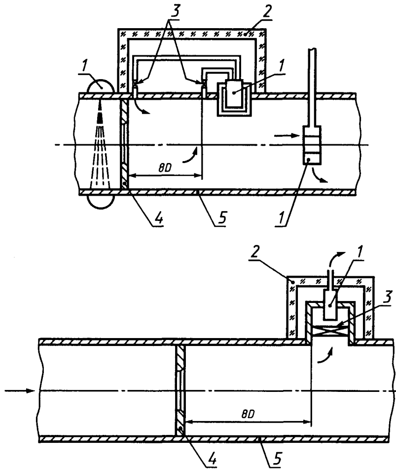
Рисунок 12 — Схемы установки плотномеров
