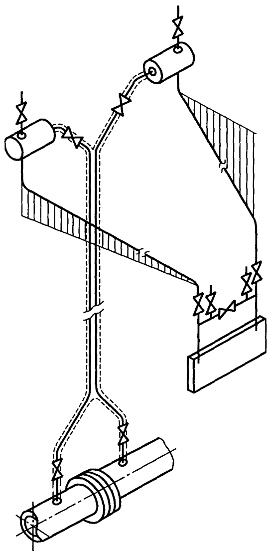
Рисунок В.7— Дифманометр над трубопроводом
