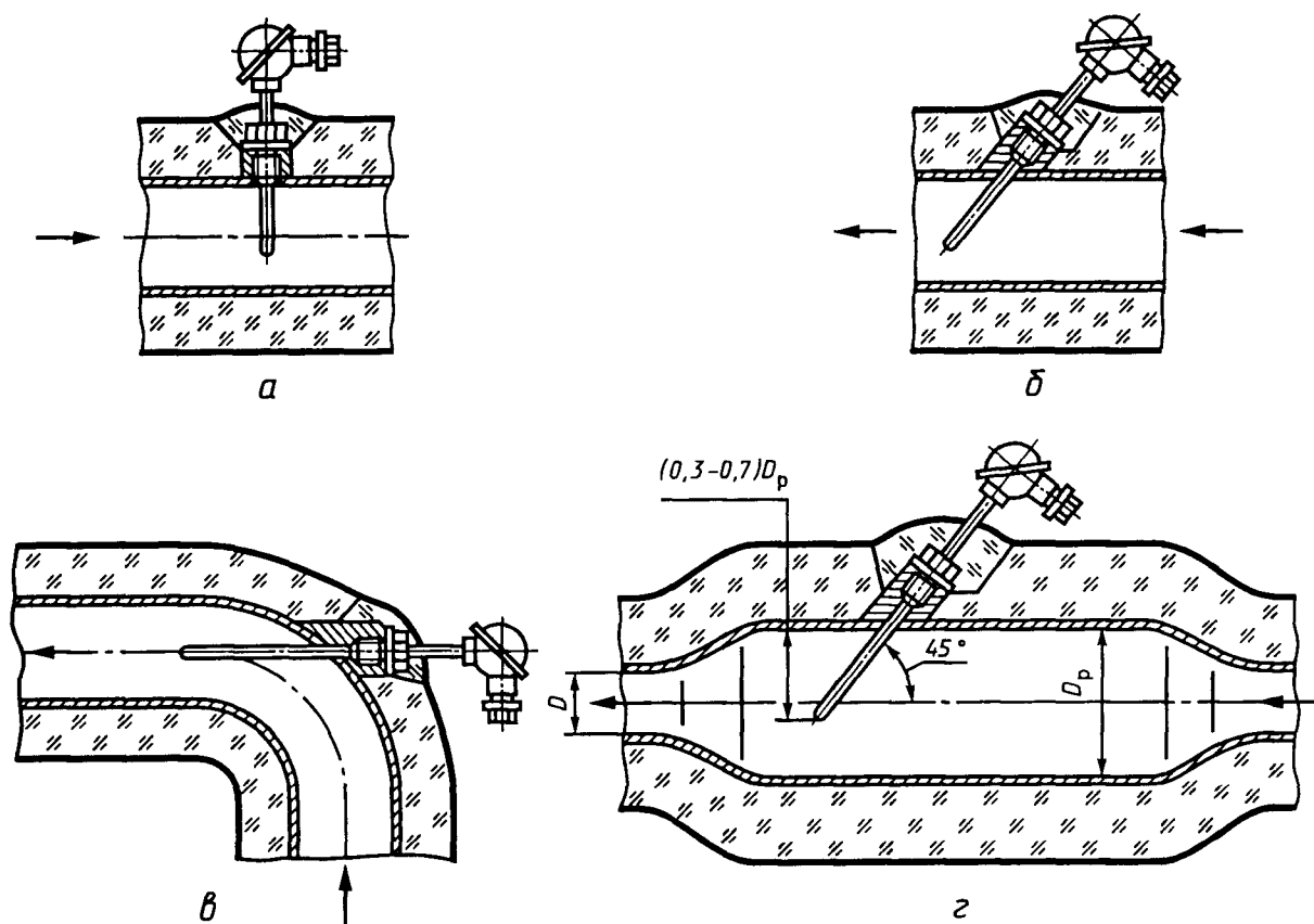
Рисунок 11— Схема установки чувствительного преобразователя термометра
