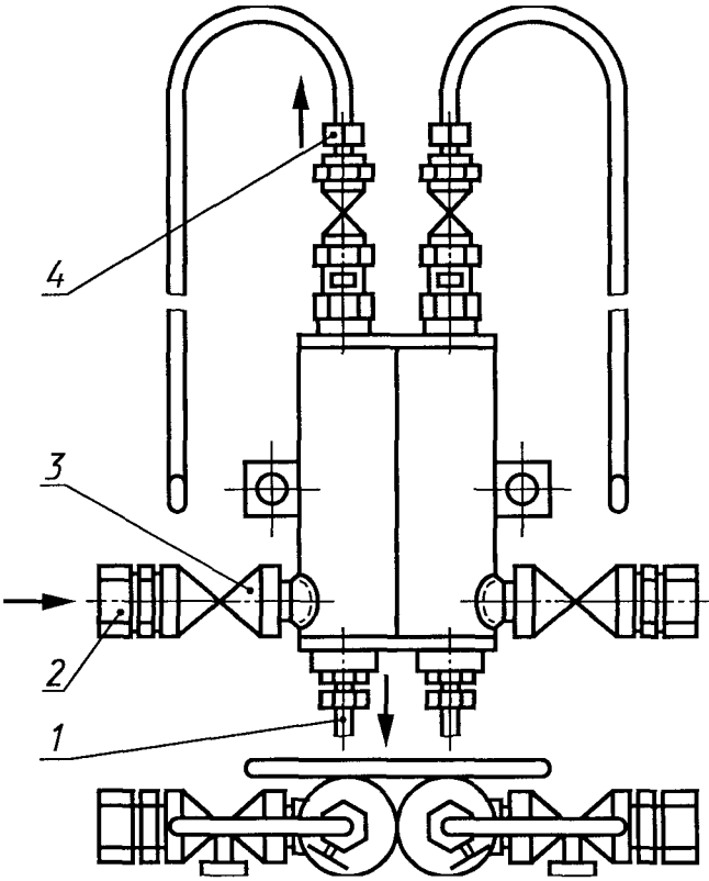
1 — выходной патрубок; 2 — входной патрубок; 3 — кран; 4 — всасывающий патрубок
