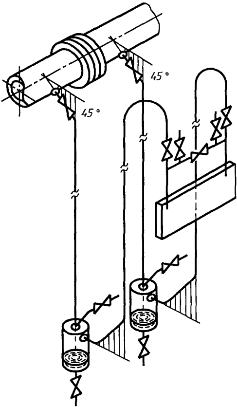
Рисунок В.10 — Дифманометр под трубопроводом (вариант)
