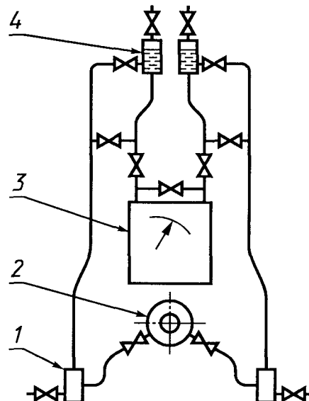
1 — отстойная камера; 2 — сужающее устройство; 3 — дифманометр; 4 — воздухо-сборник
