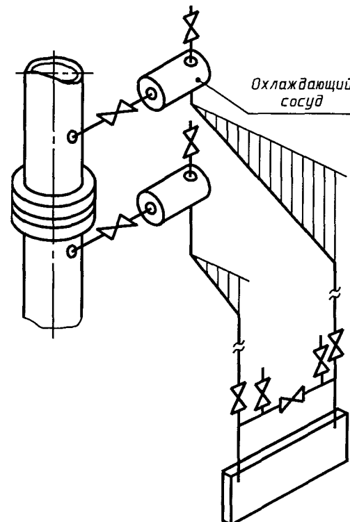
Рисунок В.17 — Вертикальный трубопровод
