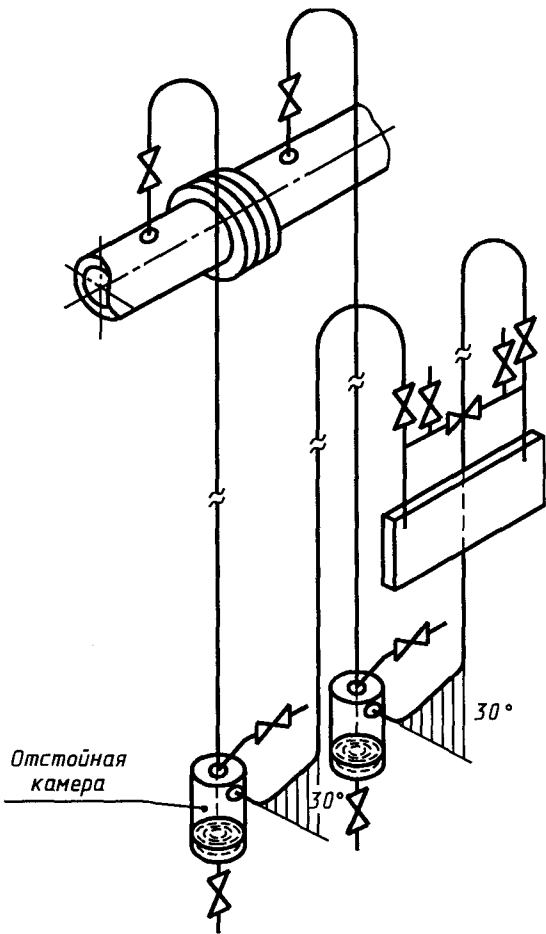
Рисунок В.9 — Дифманометр под трубопроводом
