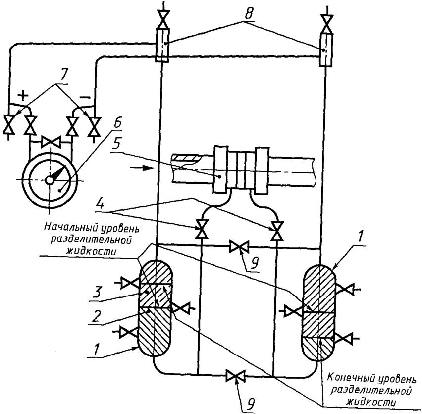
1 — разделительный сосуд; 2 — контролируемая жидкость; 3 — разделительная жидкость; 4 — запорный вентиль сужающего устройства; 5 — сужающее устройство; 6 — дифференциальный манометр; 7 — продувочный вентиль; 8 — газосборник; 9 — уравнивательный вентиль
