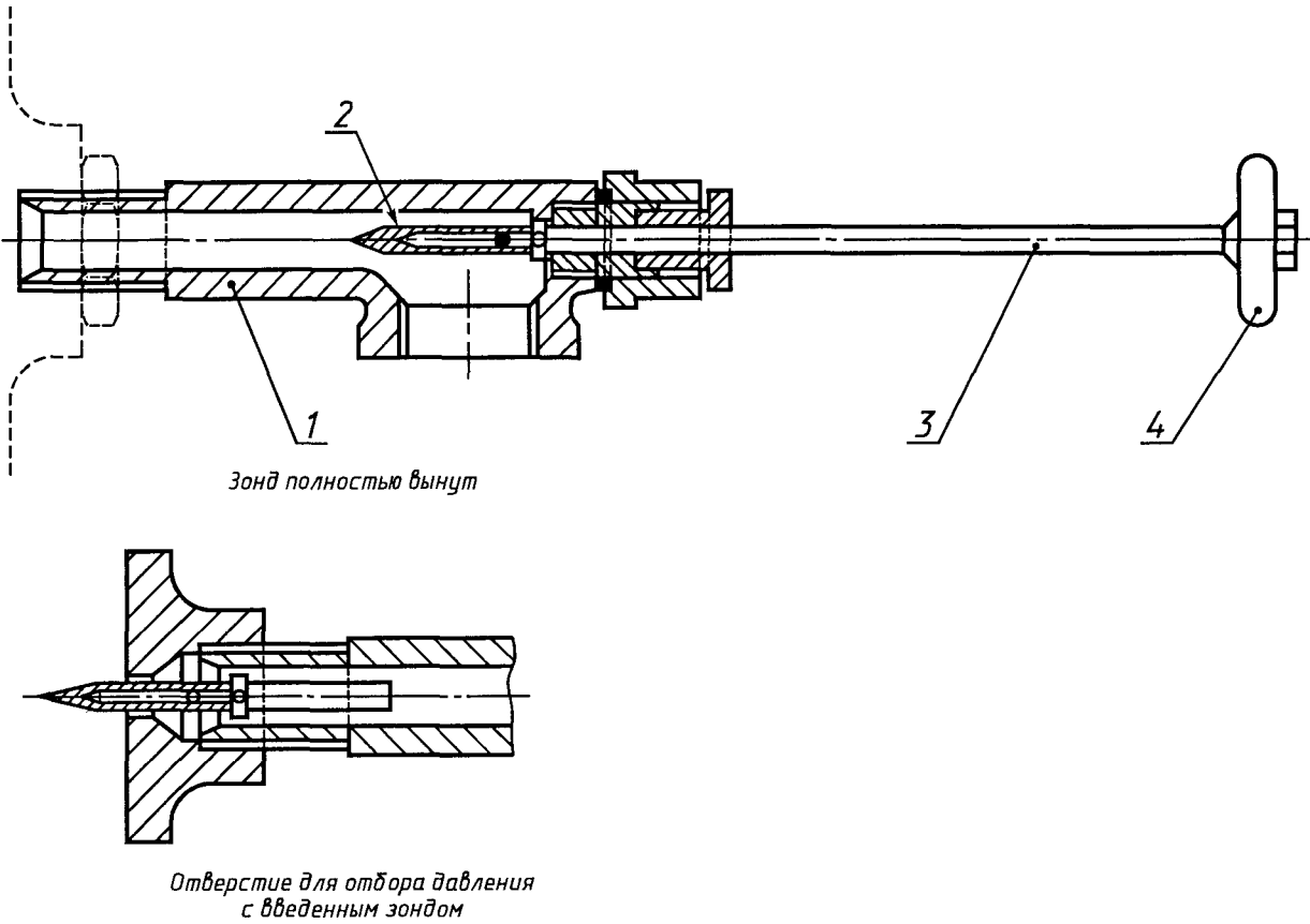
1 — корпус; 2 — головка зонда; 3 — ось зонда; 4 — рукоятка
