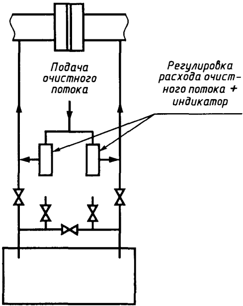
Рисунок 9 — Пример установки очистной системы
