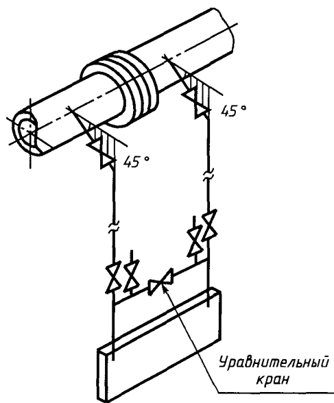
Рисунок В.15 — Дифманометр под трубопроводом
