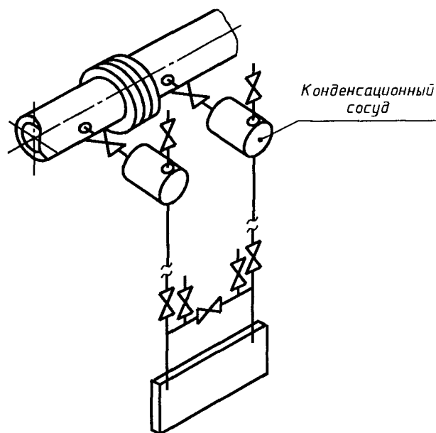
Рисунок В.5 — Дифманометр под трубопроводом
