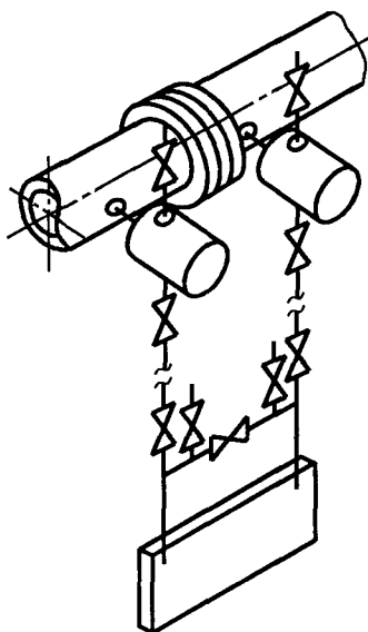
Рисунок В.6 — Дифманометр под трубопроводом (вариант)
