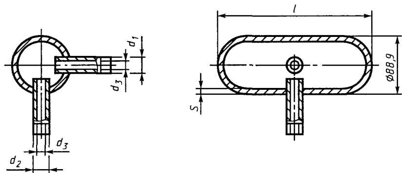
Рисунок 1 — Уравнильные сосуды, рекомендуемые [1]
