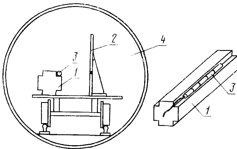
1—угловая мортира; 2—отражательная стенка; 3—заряд испытуемого ВВ; 4—штрек
