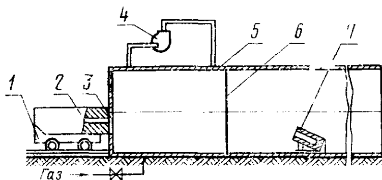
1—тележка; 2—канальная мортira; 3—люк штрека; 4—вентилятор; 5—труба штрека; 6—диафрагма; 7— распылительная мортira
