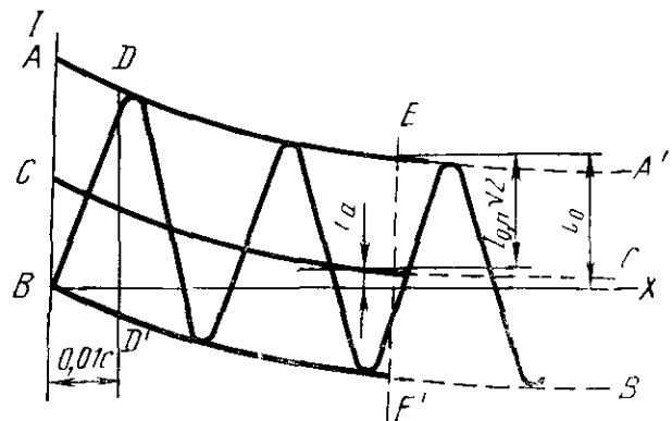
Периодическая и апериодическая составляющие тока короткого замыкания
