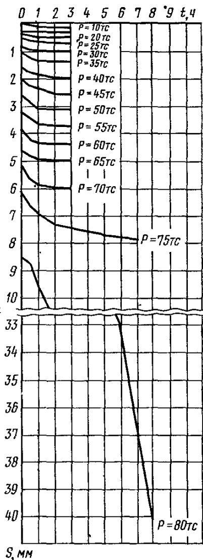
График изменения осадки сваи S во времени t (по ступеням нагрузки)
