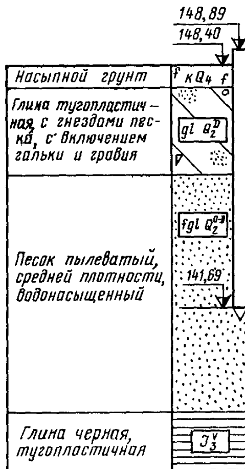
Геологический разрез
