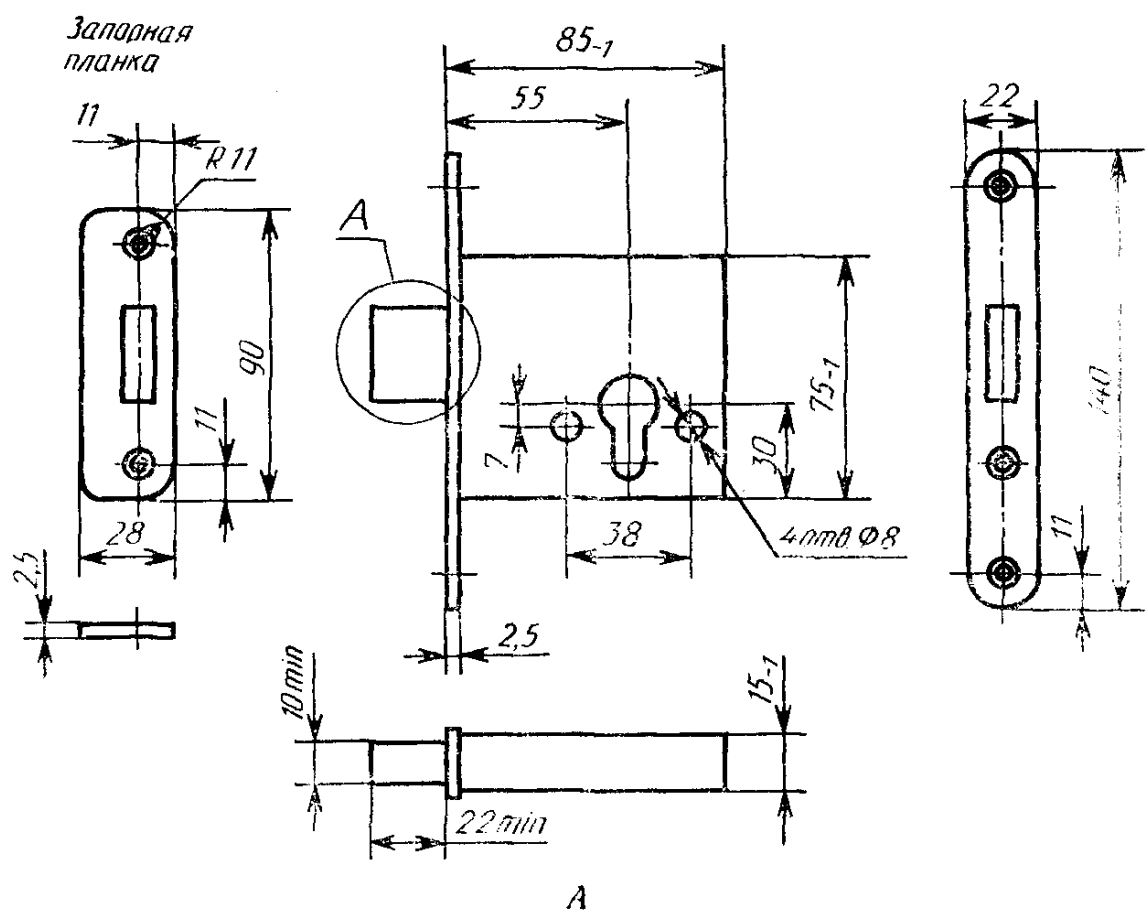
Вариант исполнения засова и запорной планки
