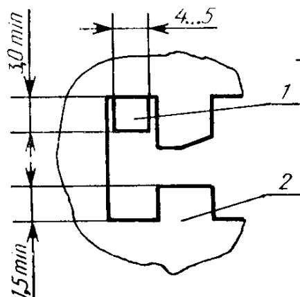
1 — это — хвостовика; 2 — сувальда Черт. 47
