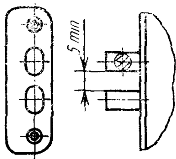
Вариант исполнения засова и запорной планки
