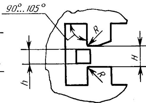
1 — это — хвостовика; 2 — сувальда Черт. 47
