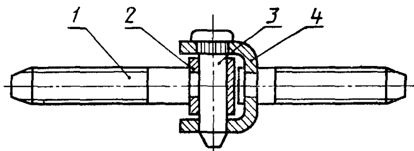
1 — стержень, 2 — втулка; 3 — ось; 4 — скоба
