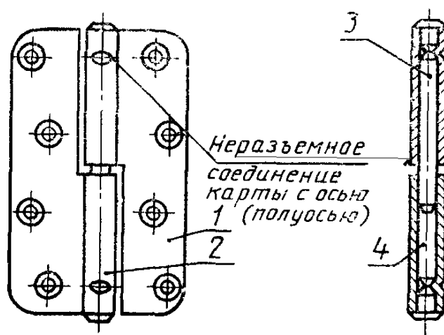
1 — карта; 2 — трубка; 3 — ось; 4 — полуось
