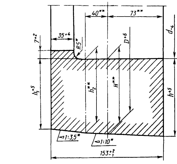
Круг катания
