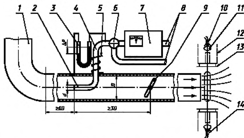
1 — выпускная труба; 2 — газоотборный зонд; 3 — дифференциальный манометр; 4 — газоподводящая труба; 5 — теплообменник; 6 — байпасный клапан; 7 — дымомер частично-поточный; 8 — газоподводящие трубы; 9 — регулируемая заслонка; 10 — источник света; 11 — собирающая линза; 12 — дымомер полнопоточный (на срезе выпускной трубы); 13 — разделительная перегородка; 14 — приемник света
