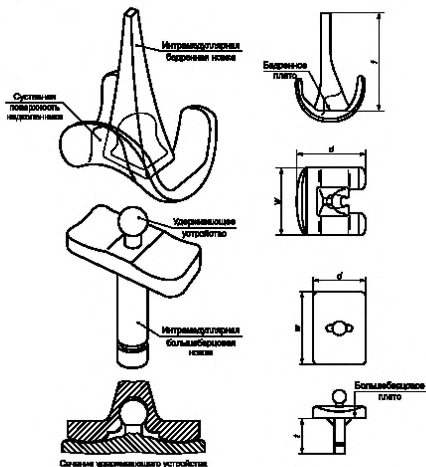
Рисунок 5 — Типичный частично связанный тотальный эндопротез коленного сустава с интратрубулярными ножками (см. примечание к разделу 4)
