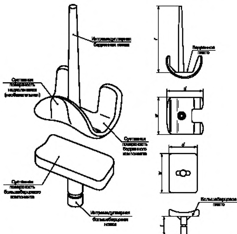
Рисунок 2 — Типичный свободный двухмыщелковый тотальный эндопротез коленного сустава с интрамедуллярными ножками (см. примечание к разделу 4)
