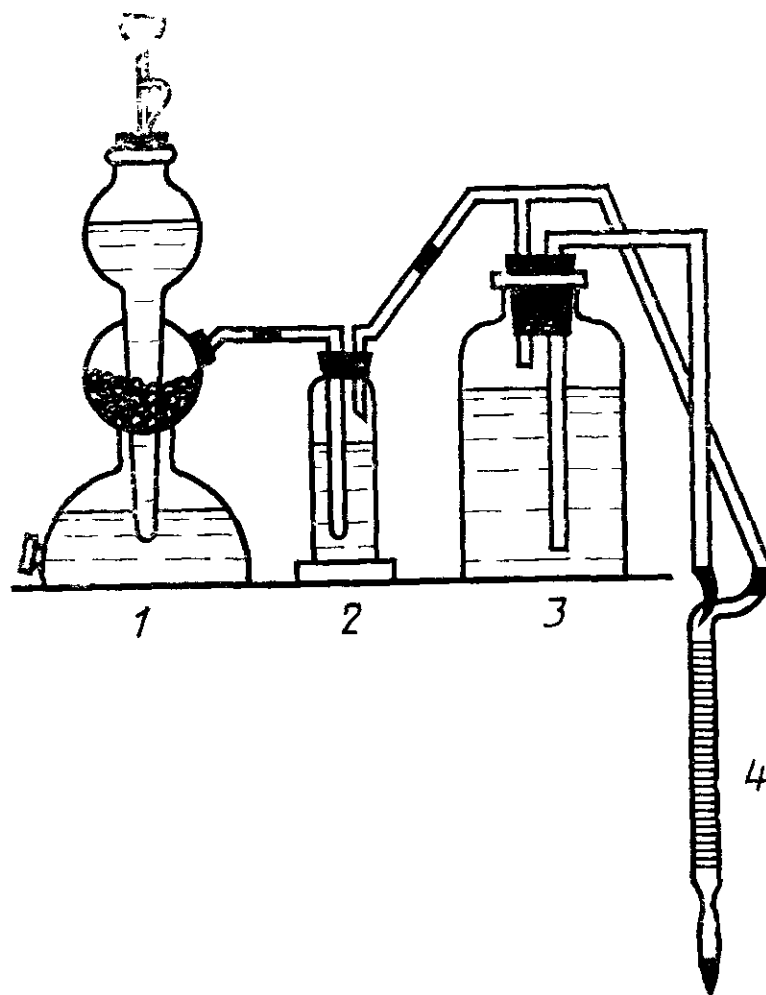
1—аппарат Киппа; 2—промывалка для газа, заполненная раствором сернокислого титана (III) 50 г/дм³; 3—сосуд с рабочим раствором, 4—бюретка.
