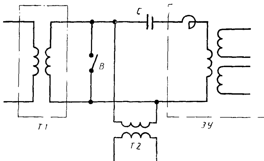
T1 — питающий трансформатор; C — конденсатор отбора мощности емкостного трансформатора; T2 — трансформатор напряжения; ZU — электромагнитное устройство емкостного трансформатора
