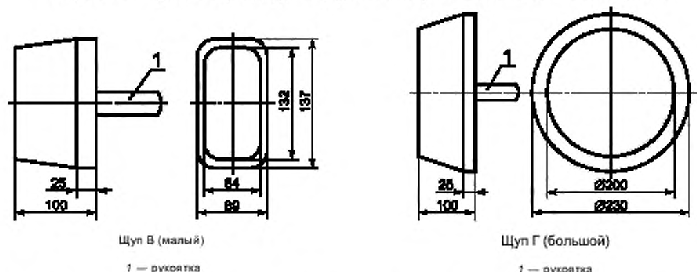
Рисунок Г.2 — Щуп В (малый) для определения застревания головы или шеи в отверстиях
