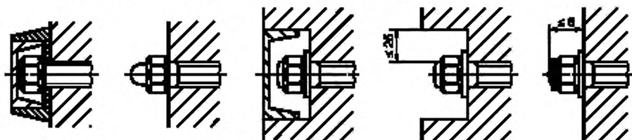
Рисунок 4 — Защита болтовых соединений
