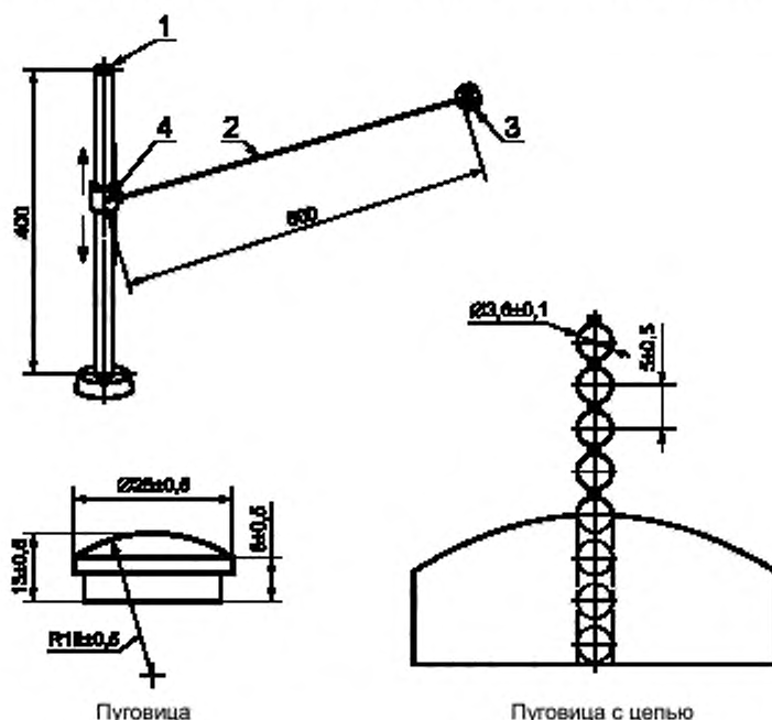
1 — стойка; 2 — петля; 3 — пуговица из полимерного материала; 4 — втулка; R — радиус лицевой поверхности пуговицы
