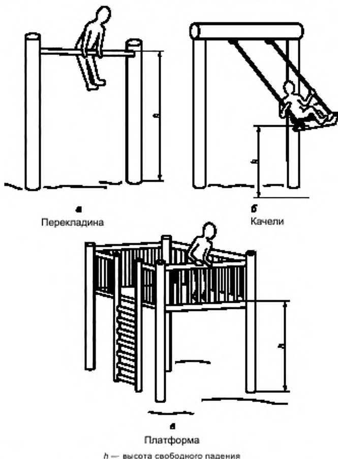
Рисунок 13 — Высота свободного падения h для различного оборудования
