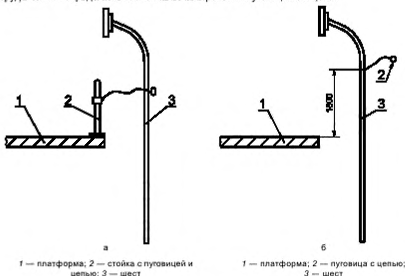
Рисунок Г.11 — Испытания шеста
