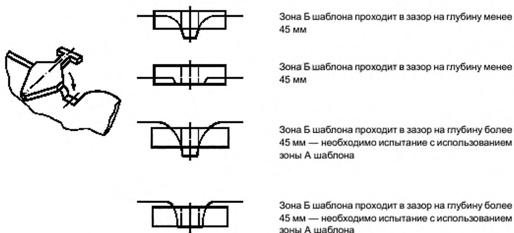
Рисунок Г.5 — Испытания V-образных зазоров с использованием зоны Б шаблона
