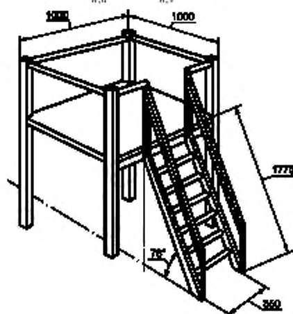
Рисунок А.1 — Платформа с лестницей
