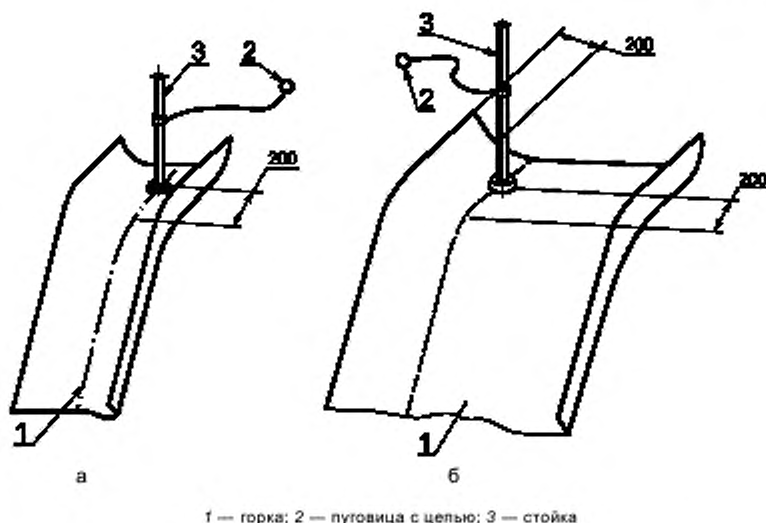
Рисунок Г.10 — Размещение испытательного устройства на горке
