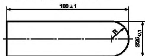
Рисунок Г.13 — Стержень-палец Б (большой)
