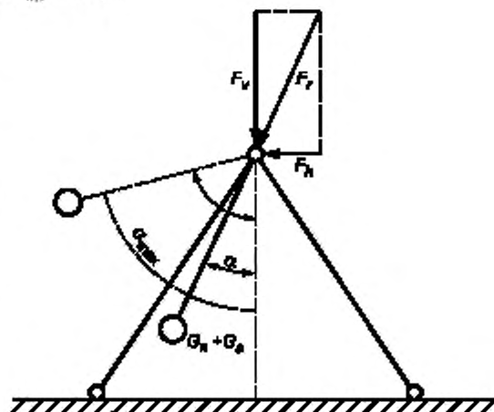
F_h — горизонтальная нагрузка на узел; F_v — вертикальная нагрузка на узел; F_r — нагрузка на узел; G_s — масса качелей; G_n — масса детей; \alpha — угол отклонения качелей; \alpha_{\max} — максимальный угол отклонения качелей 80^\circ .
