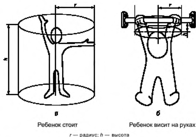
Рисунок 11 — Размеры цилиндра для определения зоны безопасности
