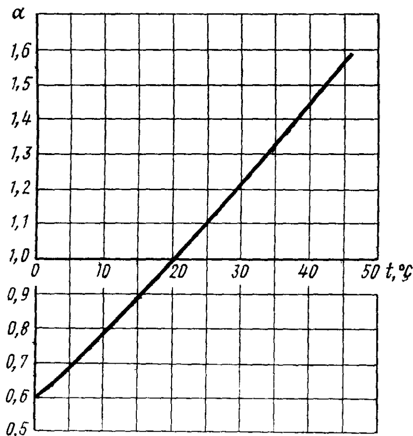
Черт. 11
