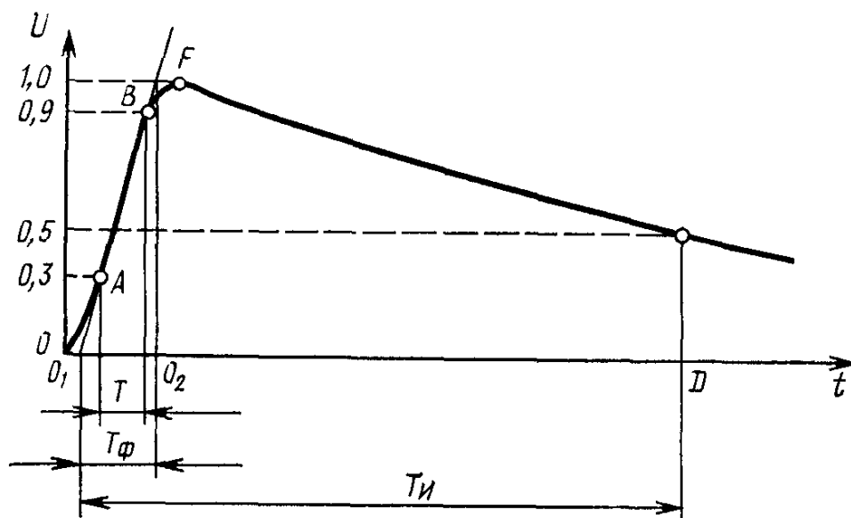
Полный грозовой импульс
