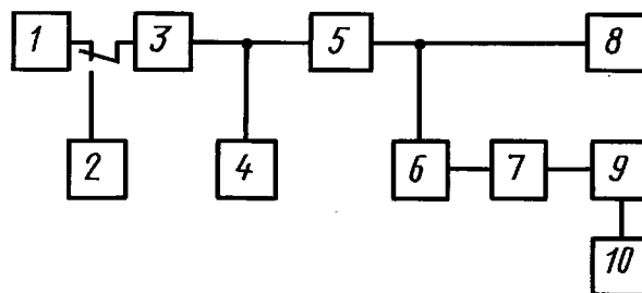
Схема измерения ширины контрольной полосы частот для излучений классов А3А, А3В, А3Н и А3Л
