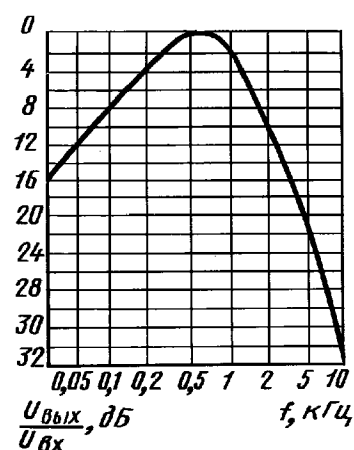
Характеристика формирующего фильтра
