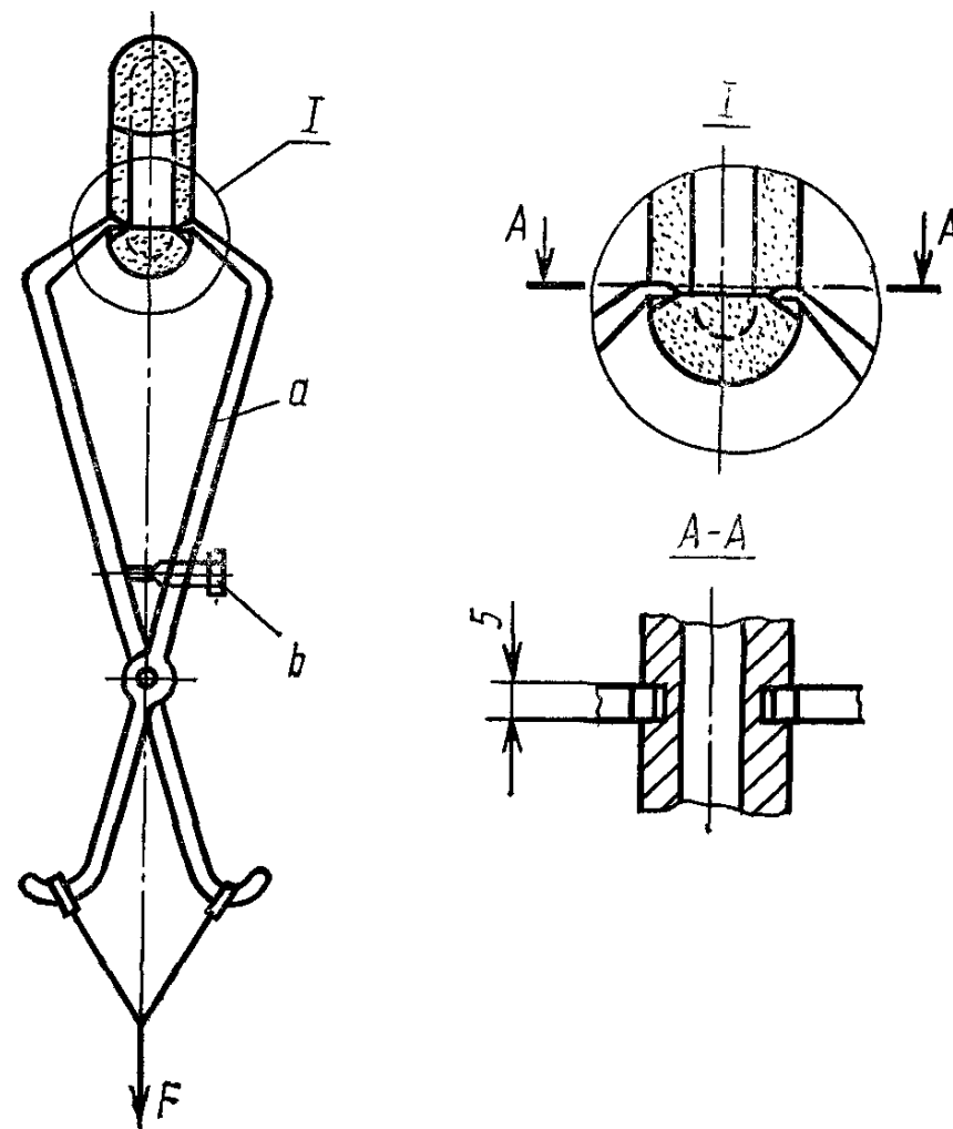
Черт. 2
