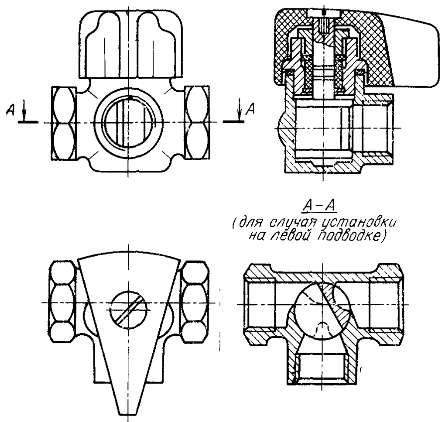
Кран регулирующий проходной с дросельным регулирующим устройством
