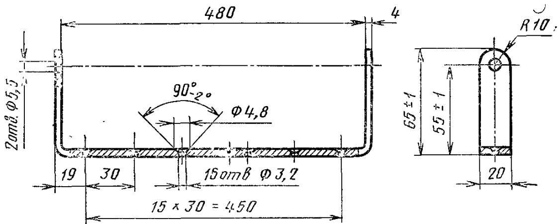
Кронштейн
