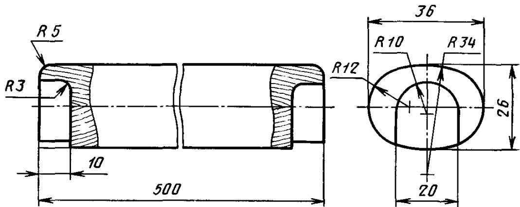
Ручка
