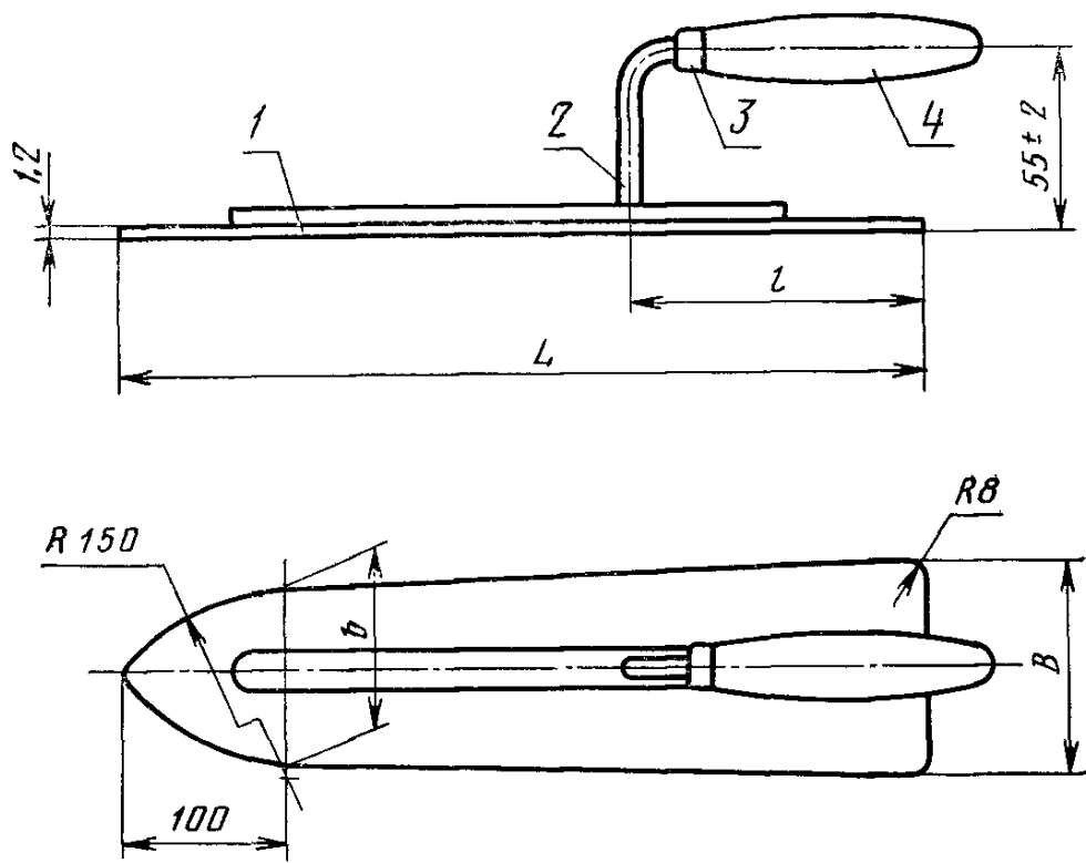
1—полотно; 2—кронштейн; 3—колпачок; 4—ручка
