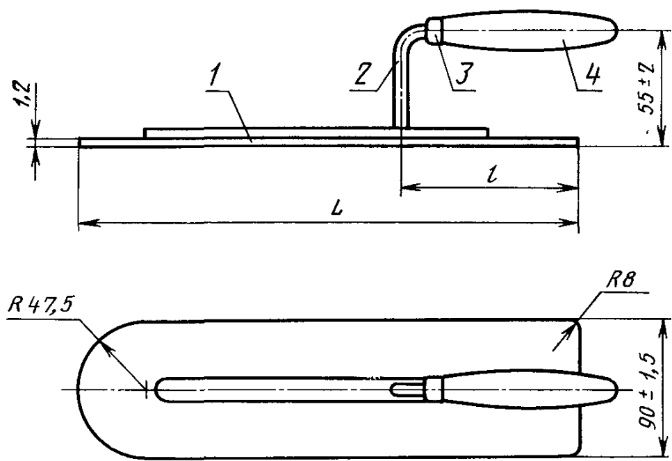
1—полотно; 2—кронштейн; 3—колпачок, 4—ручка
