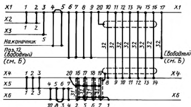
Провод поз. 30, кроме указанных особо.
